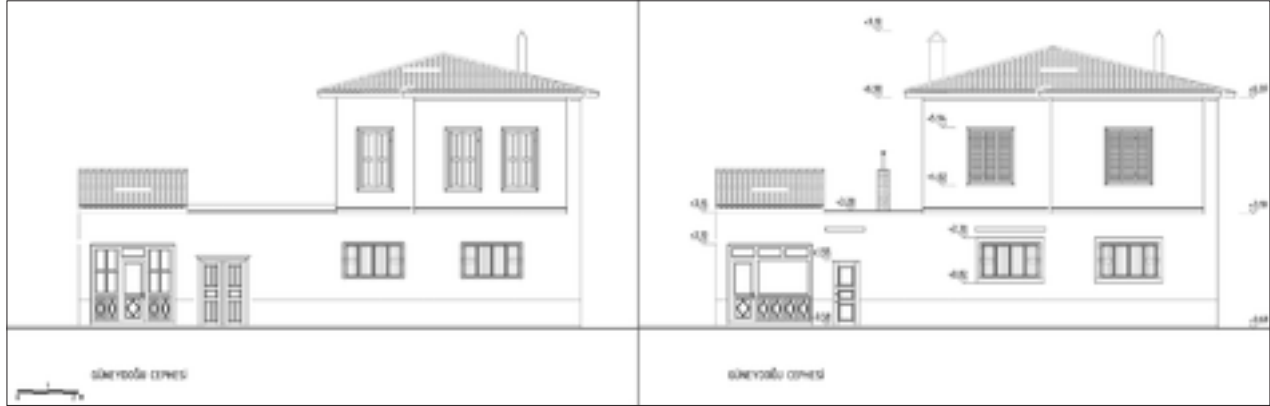
Şekil 19: Güneydoğu (Cumhuriyet Caddesi) cephesi I. ve II. dönem restitüsyon önerileri.
