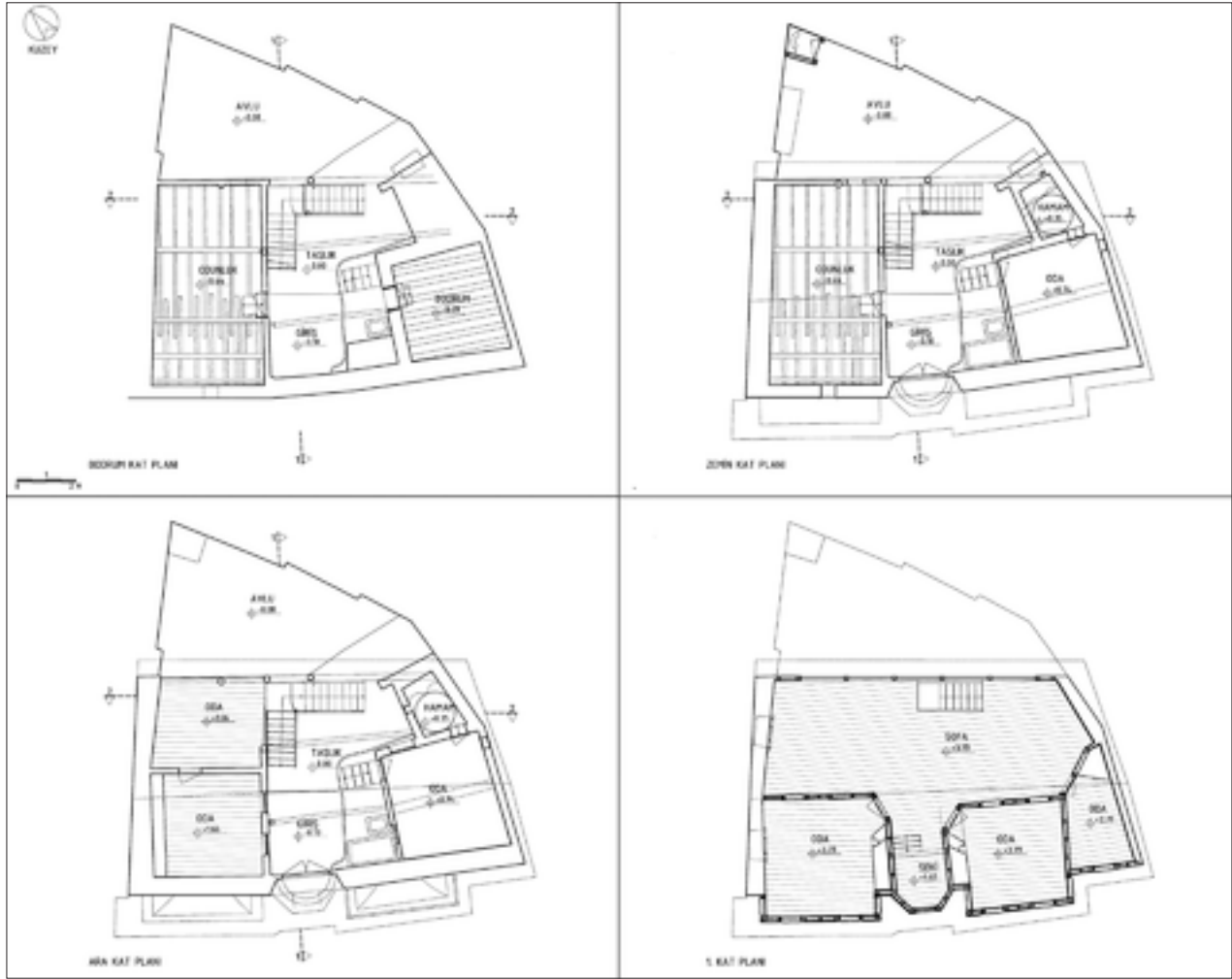
Şekil 16: I. Dönem restitüsyonu kat planları.
