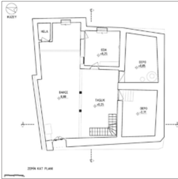
Şekil 11: Zemin kat planı restitüsyon önerisi.
