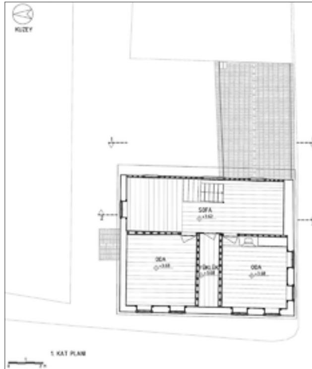
Şekil 21: Restorasyon kat planları - birinci kat planı.
