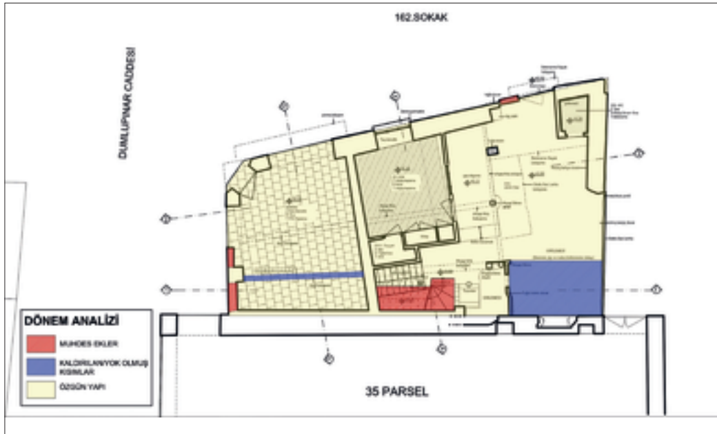
Şekil 9: Zemin kat planı dönem analizi.
