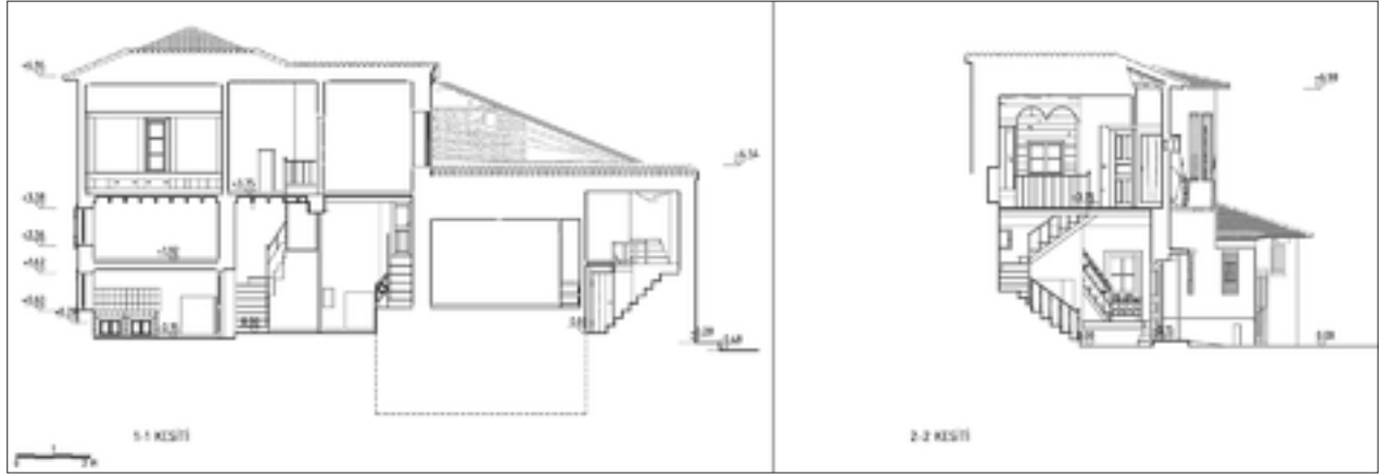
Şekil 9: Rölöve Enine ve boyuna kesit.
