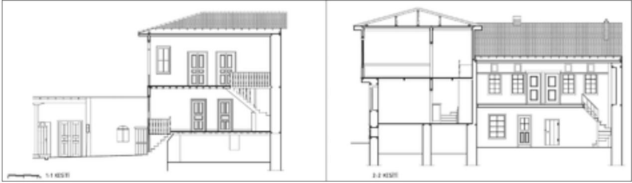
Şekil 12: Restitüsyon enine ve boyuna kesit
