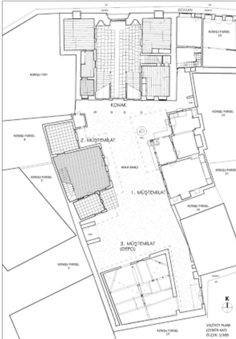
Şekil 2: Vaziyet planı.
