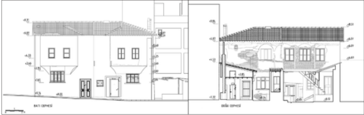
Şekil 14: 232. Sokak ve avlu cepheleri rölöveleri.
