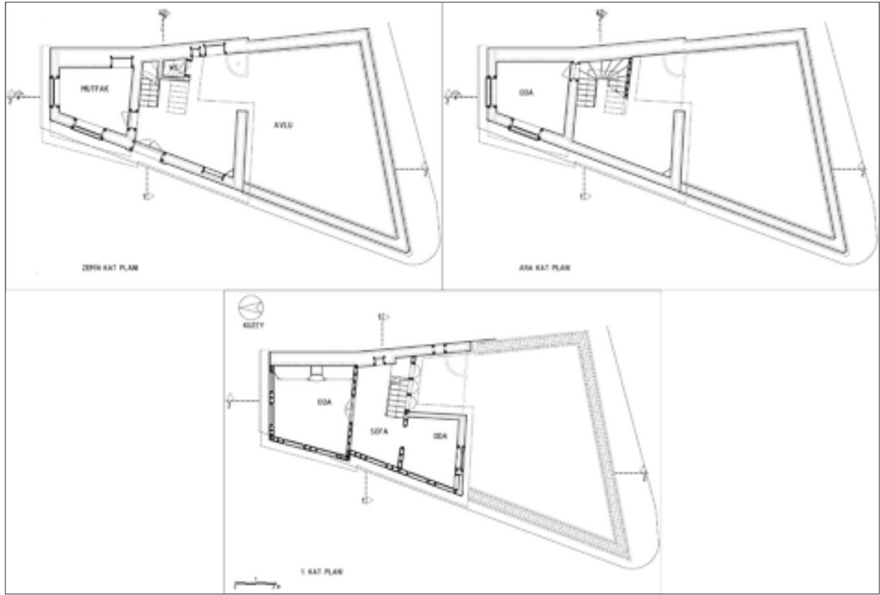
Şekil 11: Restitüsyon kat klanları.
