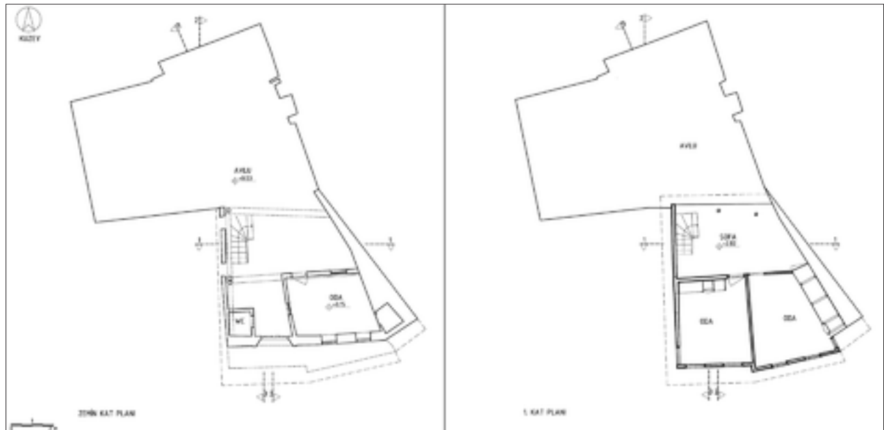
Şekil 14: Birinci dönem restitüsyon zemin ve birinci kat planları.
