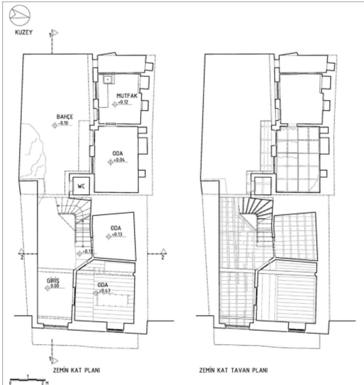
Şekil 3: Zemin kat döşeme ve tavan planları.
