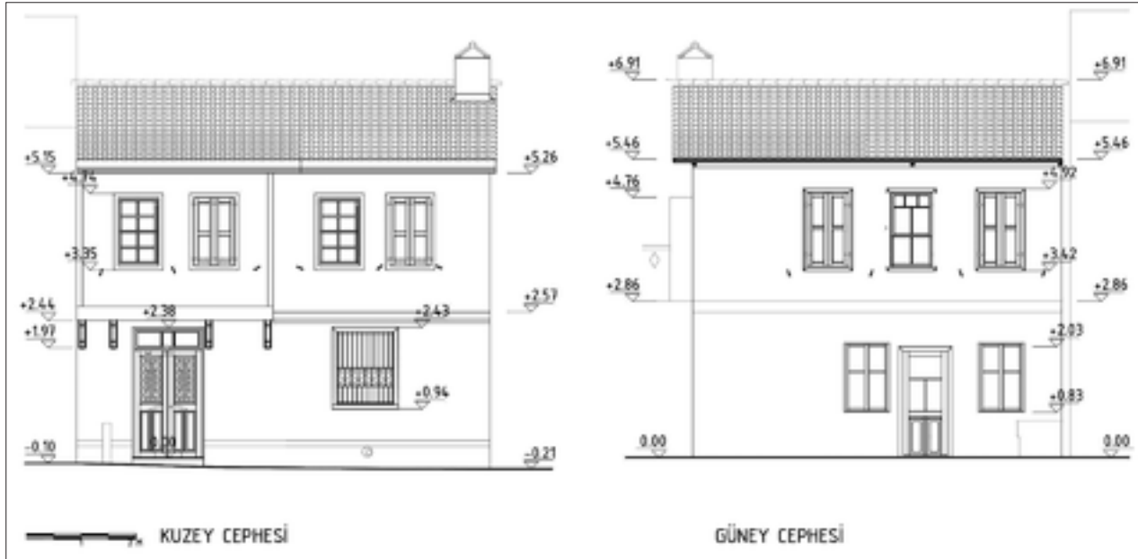
Şekil 6: Restitüsyon (1. Dönem) kuzey ve güney cephesi.
