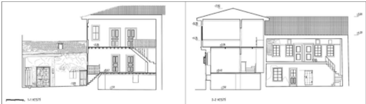
Şekil 9: Rölöve enine ve boyuna kesit
