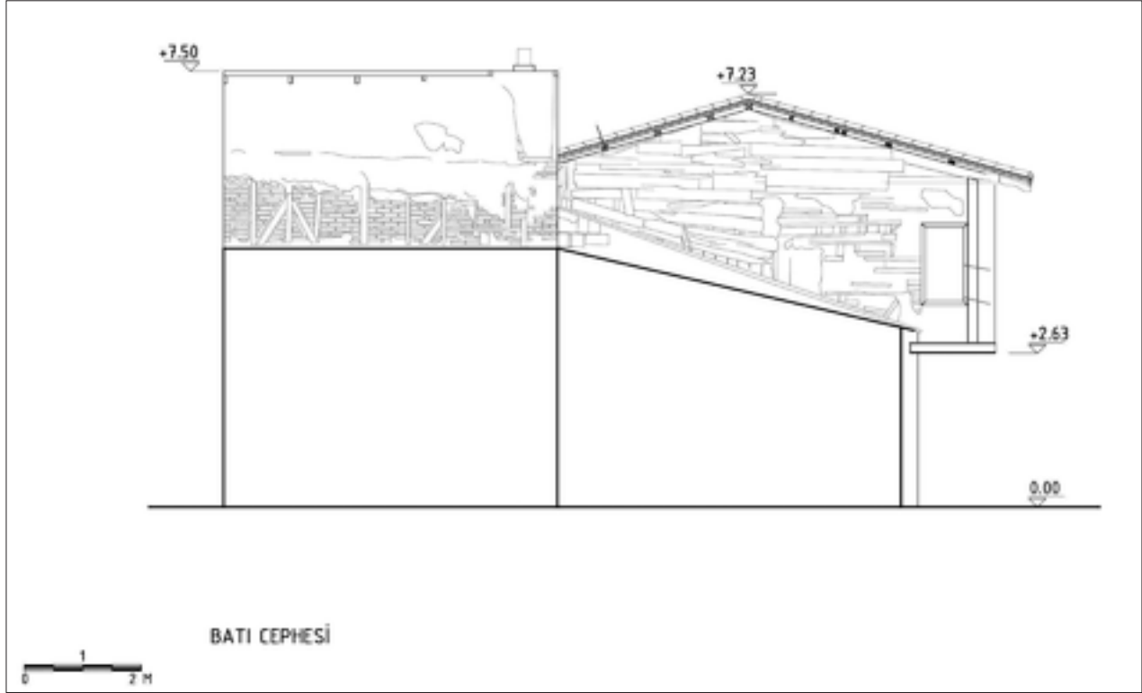
Şekil 9: Rölöve, yan cephe.
