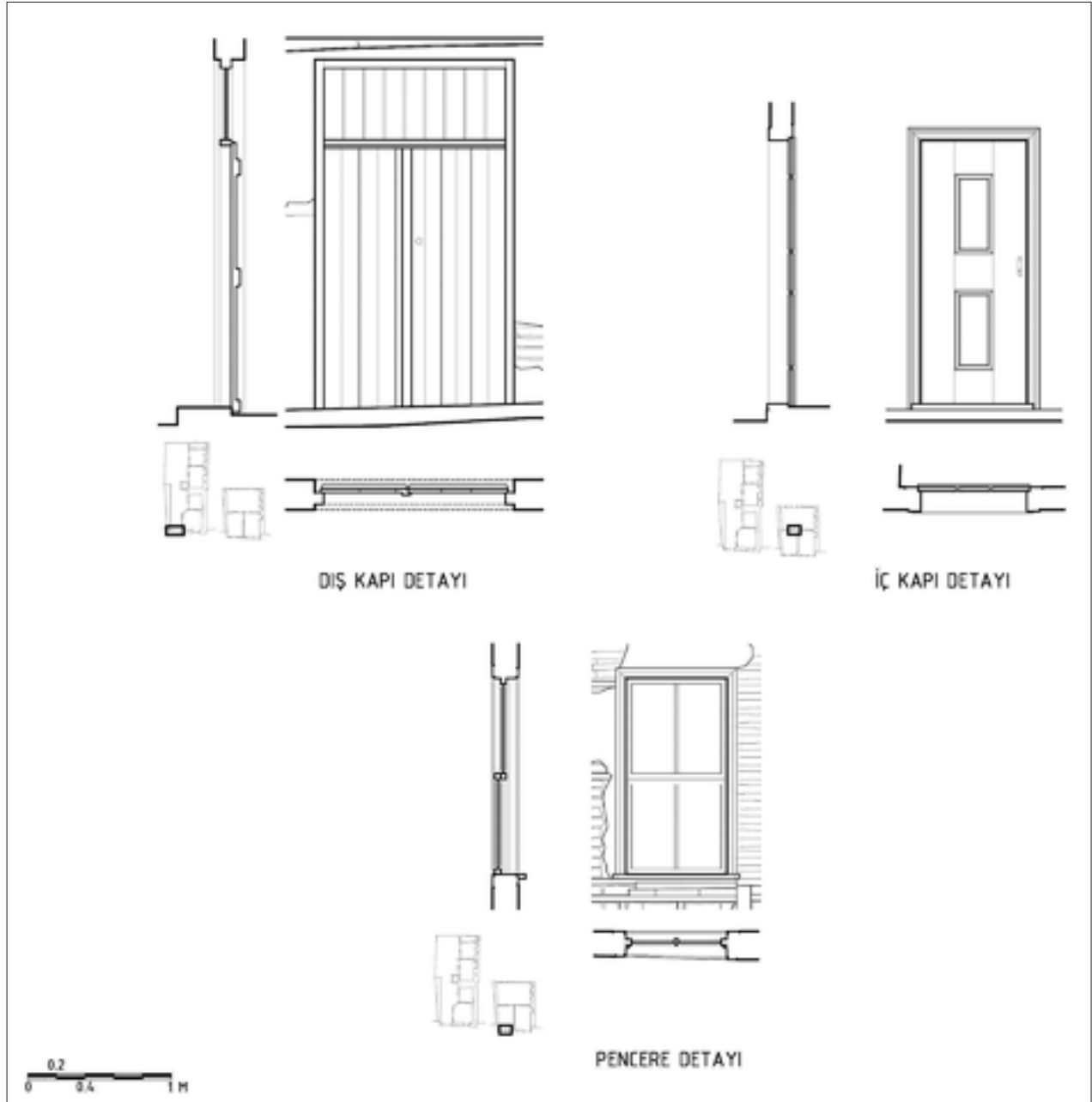
Şekil 17: Dış kapı, üst kat iç kapı ve üst kat pencere detayı.
