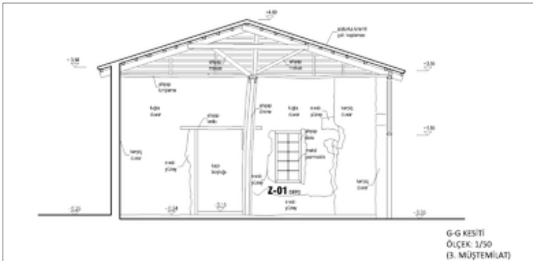
Şekil 24: Üçüncü müştemilatın kesiti (rölöve).
