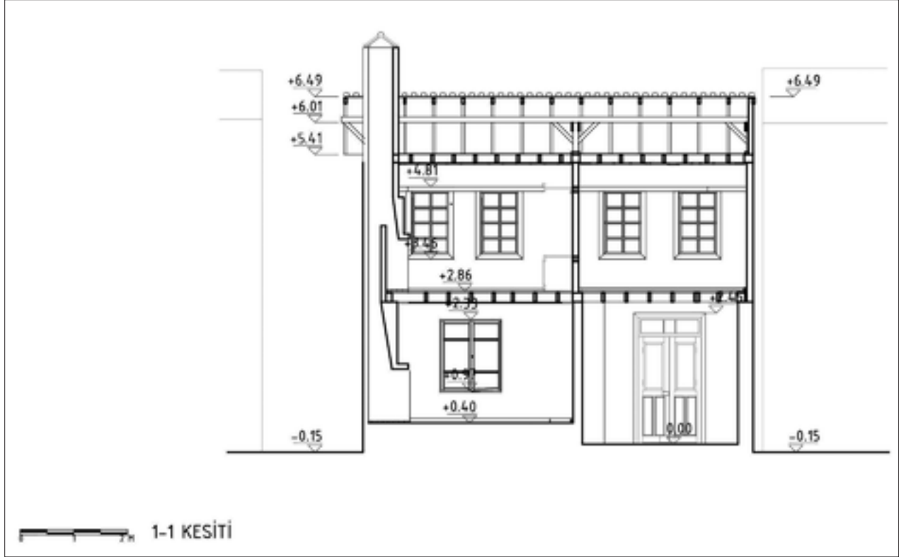
Şekil 11: Restorasyon 1-1 kesiti önerisi.
