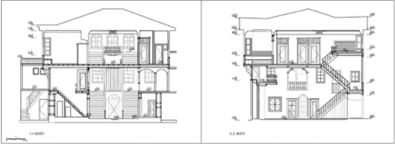
Şekil 16: Restorasyon önerisi kesitleri.
