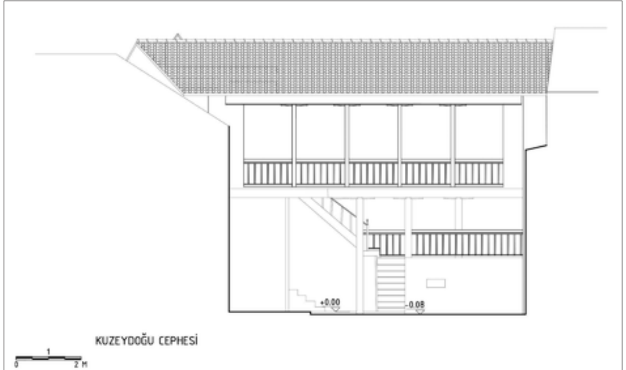
Şekil 18: I. Dönem restitüsyonu 2-2 kesiti (kuzeydoğu cephesi).
