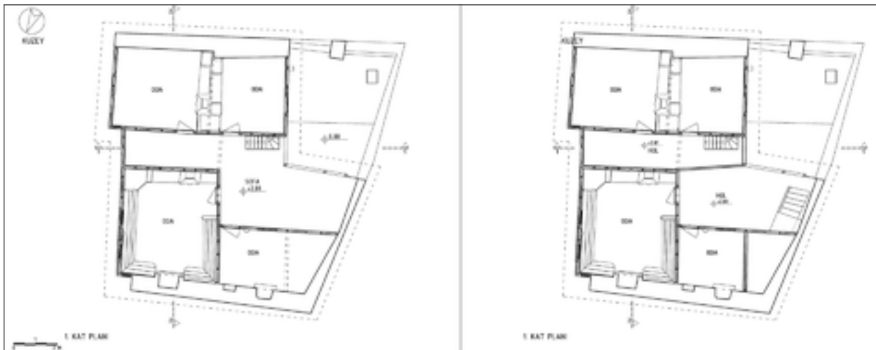
Şekil 15: 1. dönem ve 2. dönem restitüsyon önerisi 1. kat planı.
