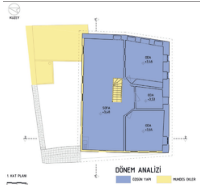
Şekil 10: Birinci kat dönem analizi.
