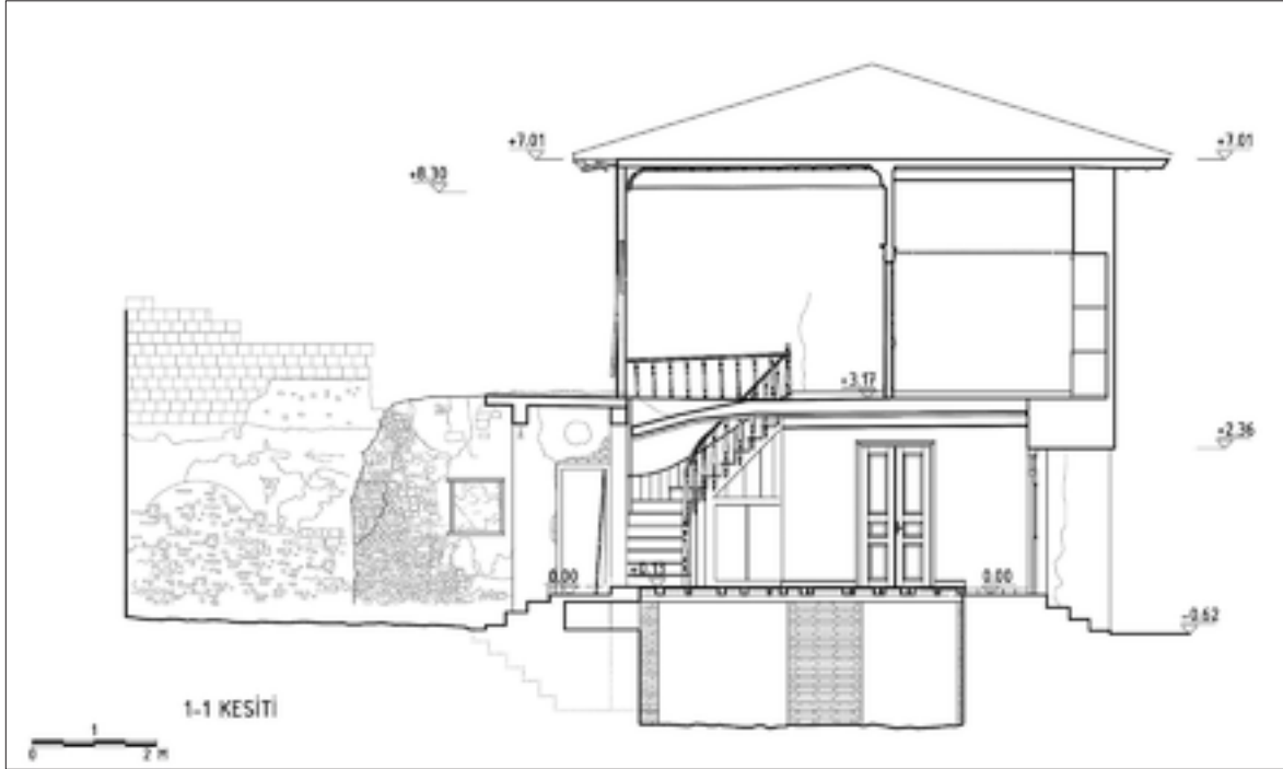
Şekil 15: 1-1 Kesiti.
