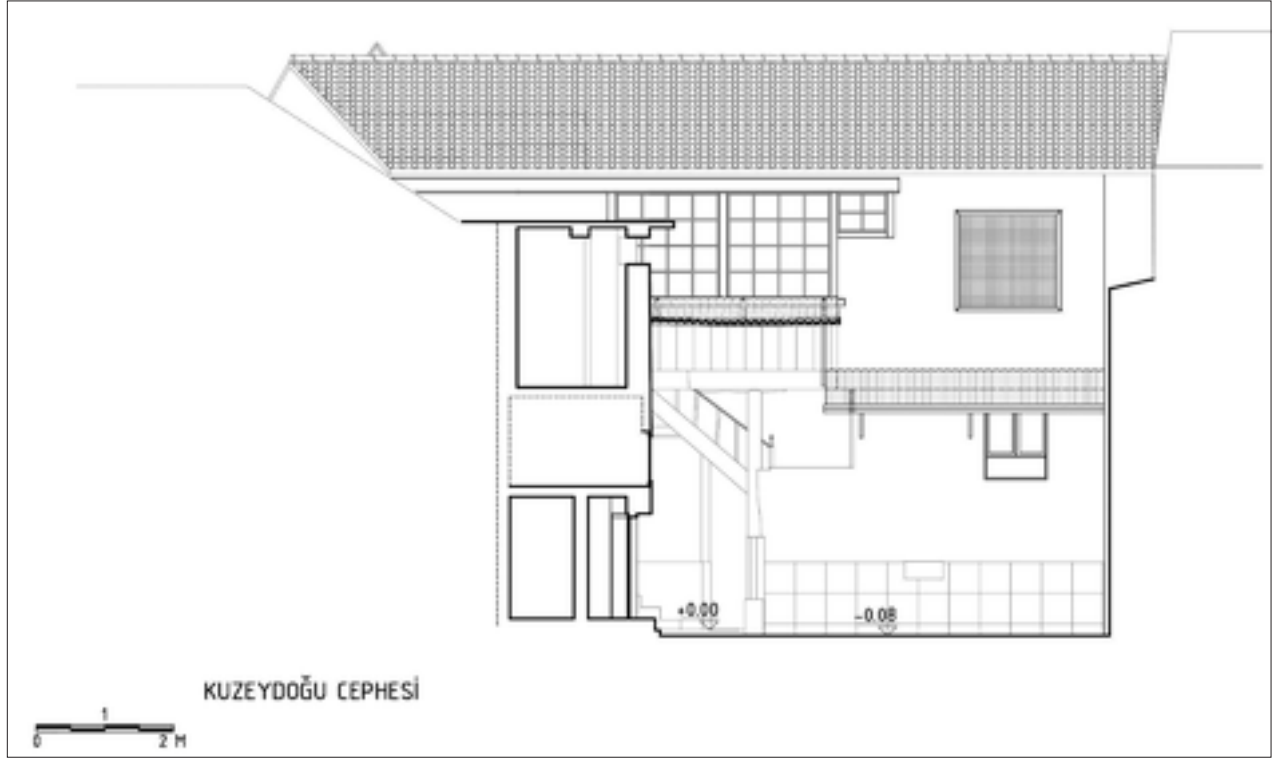
Şekil 12: Kuzeydoğu (Avlu) cephesi.
