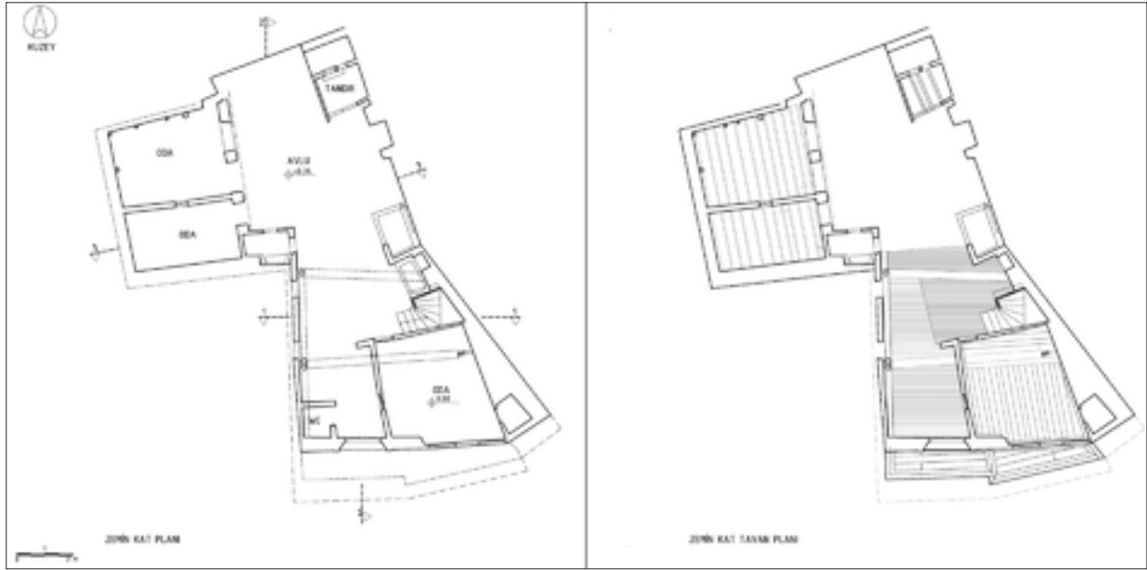
Şekil 6: Rölöve zemin kat döşeme ve tavan planı.
