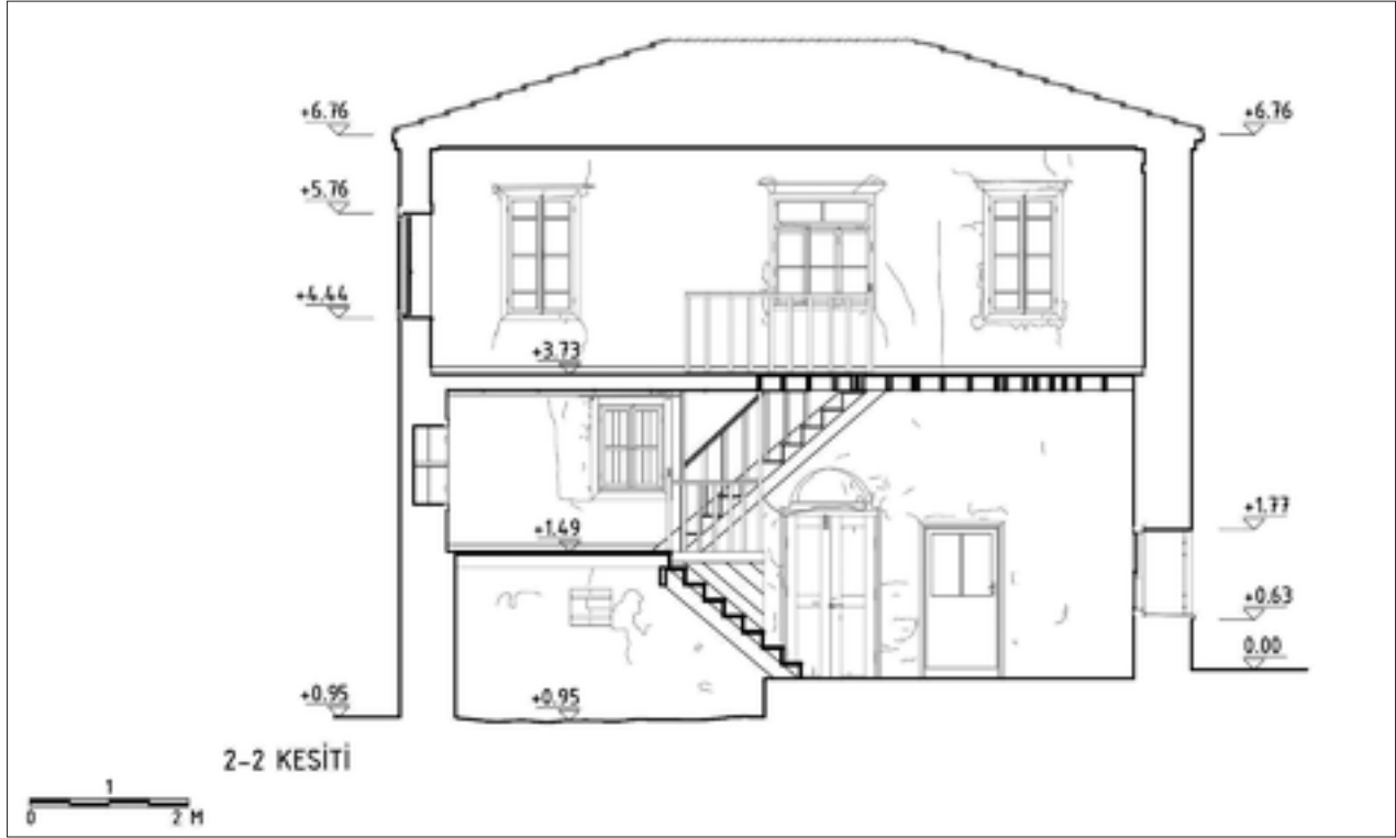
Şekil 9: Rölöve, 2-2 kesiti.
