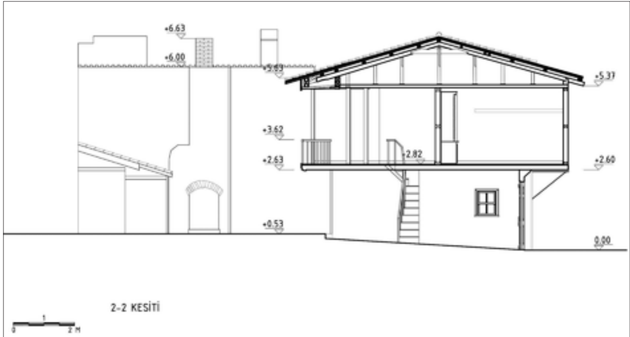
Şekil 24: Restorasyon, C-C kesiti.
