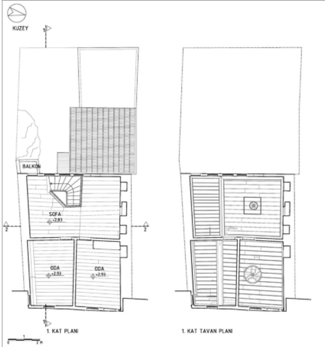
Şekil 5: Birinci kat döşeme ve tavan planları.
