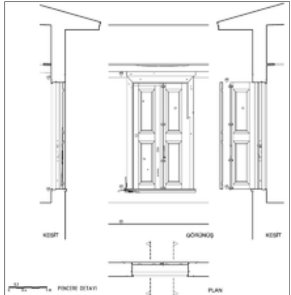
Şekil 11: Özgün pencere detayı.
