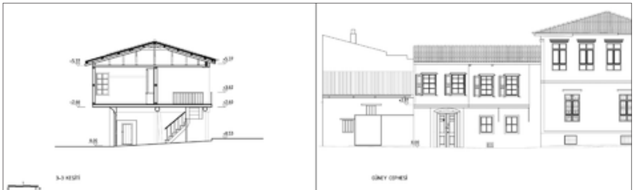
Şekil 16: Birinci dönem restitüsyon kesit ve ön cephe.
