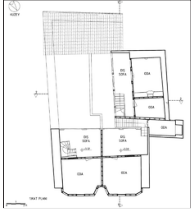
Şekil 11: İkinci dönem restitüsyonu 1. kat planı.
