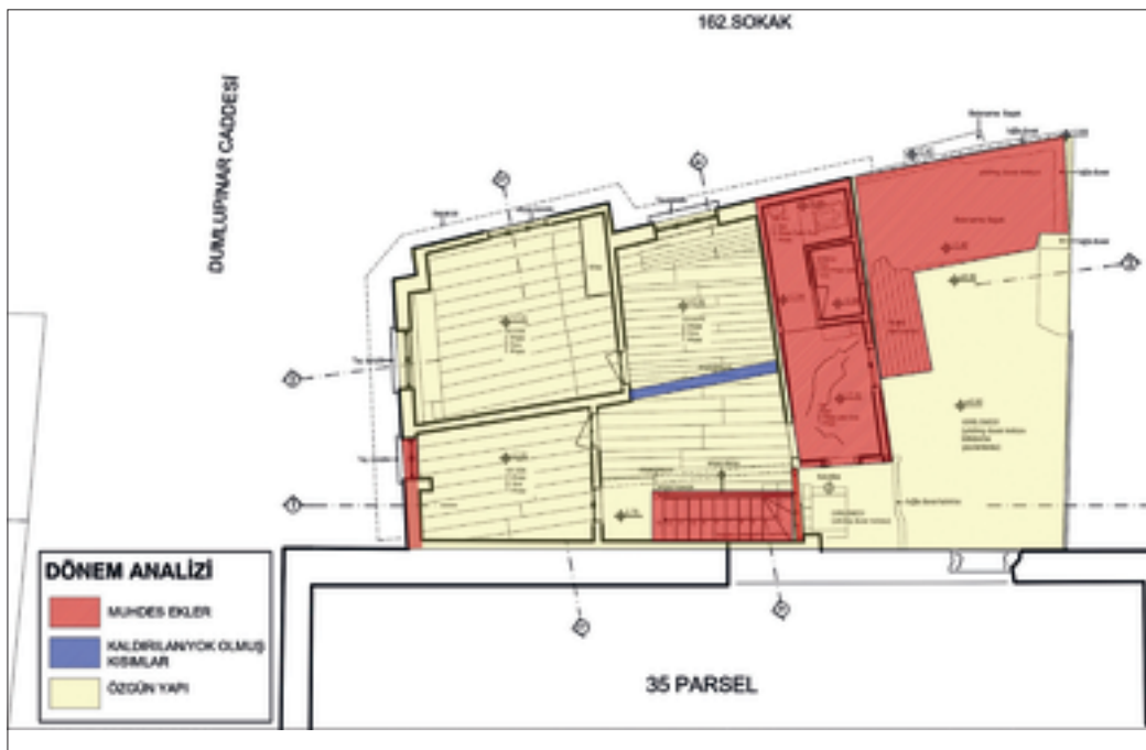
Şekil 10: Üst kat planı dönem analizi.
