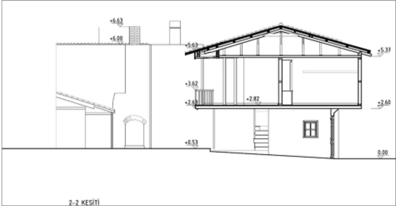
Şekil 20: Restitüsyon, 1950 ve sonrası, kesit.
