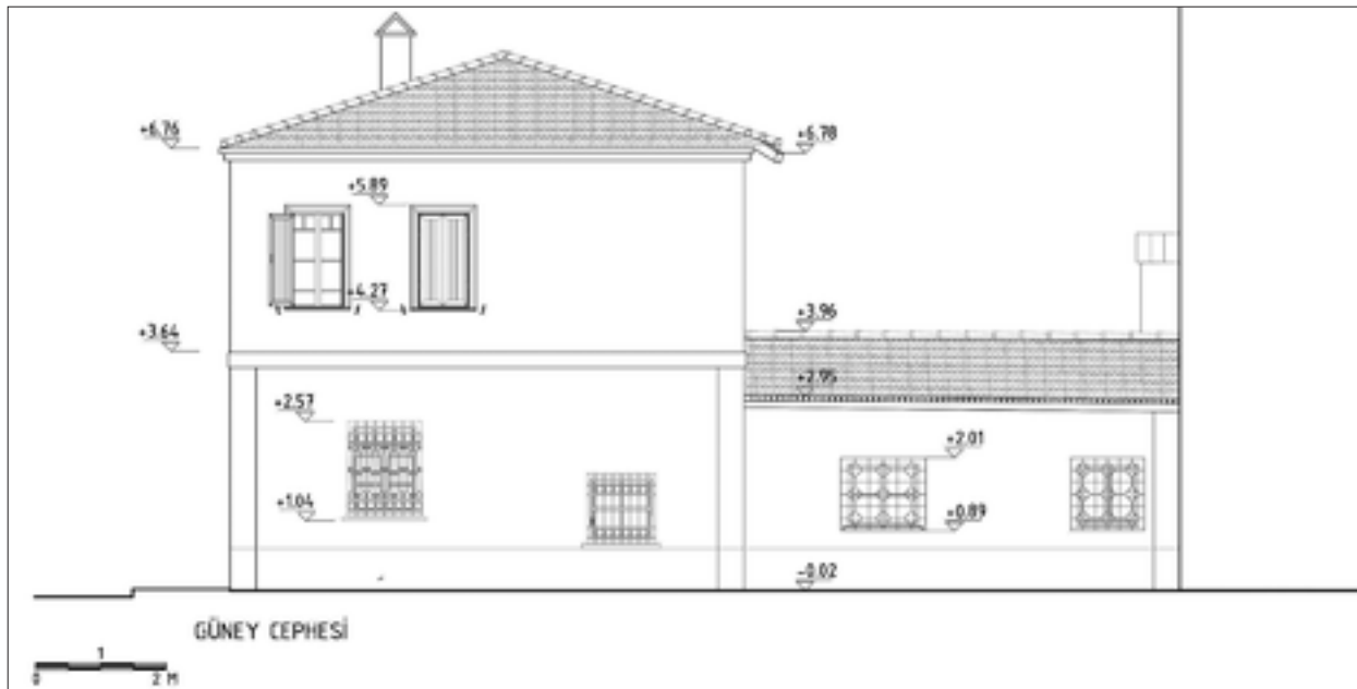
Şekil 18: Restitüsyon, yan cephe - Muhlis Kayalı Cad. görünüşü.
