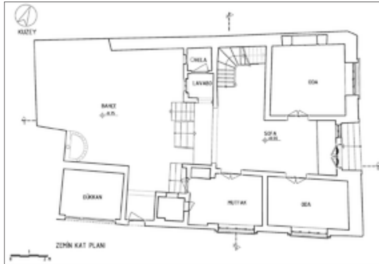
Şekil 8: Zemin kat plan rölovesi.
