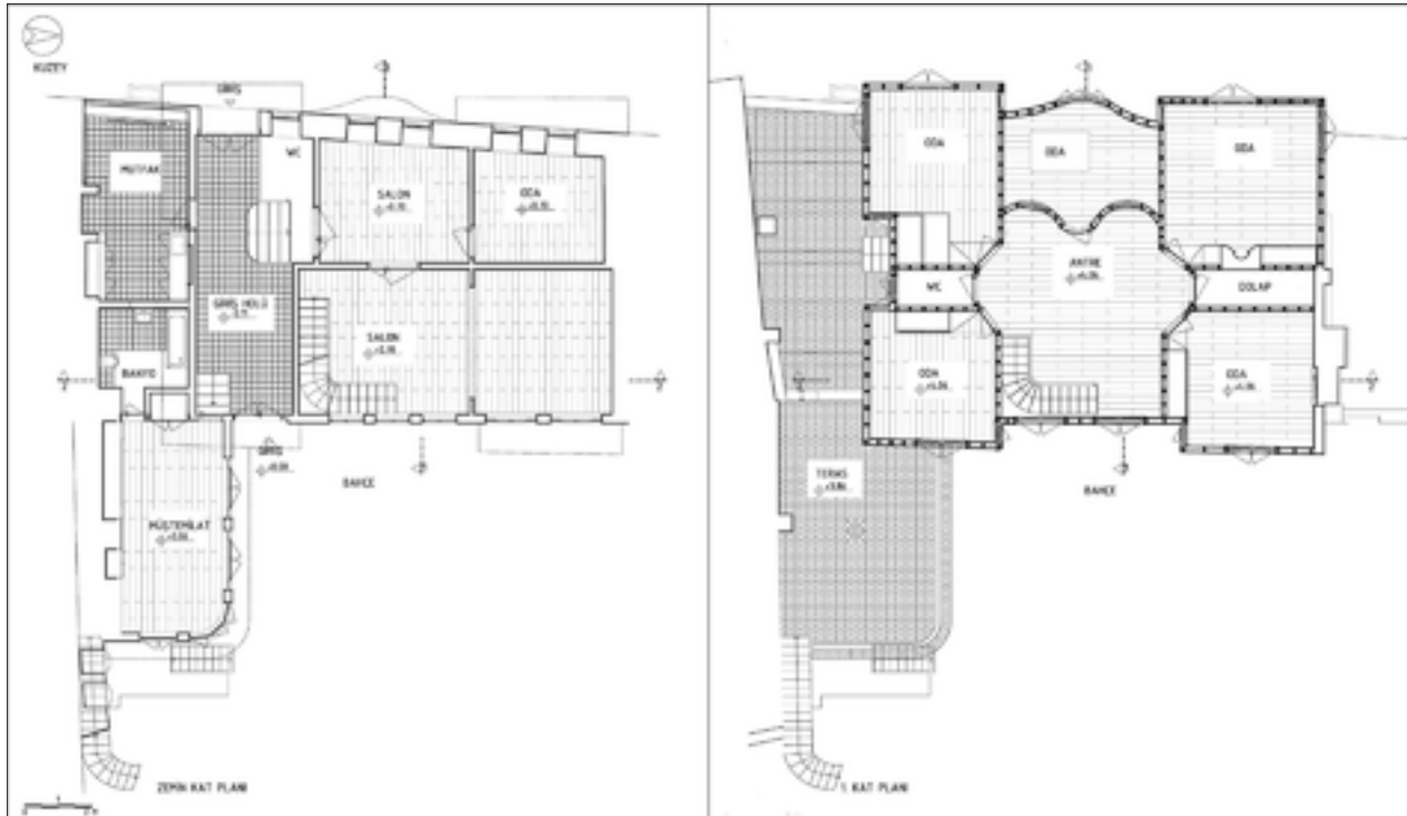
Şekil 13: İkinci dönem restitüsyon kat planları.
