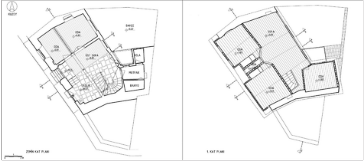
Şekil 10: 2. dönem restitüsyon kat planları.
