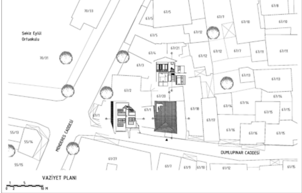
Şekil 2: Vaziyet planı.
