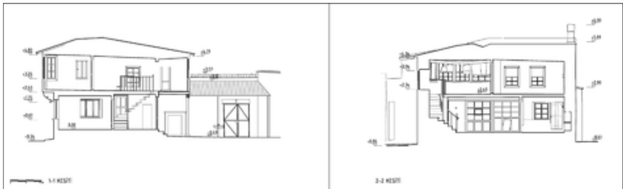
Şekil 7: Rolöve enine ve boyuna kesit.
