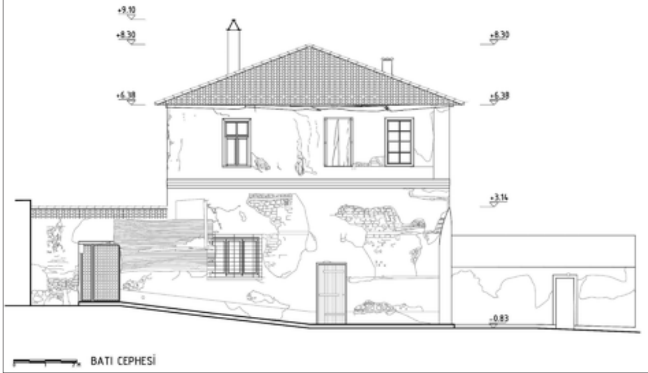
Şekil 6: Güneybatı cephesi rölövesi.
