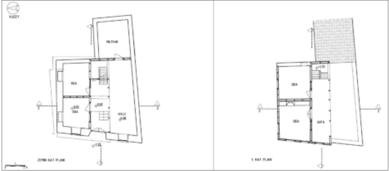
Şekil 21: Zemin ve birinci kat planları.
