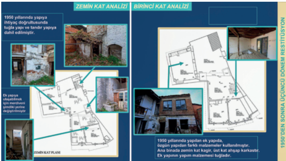
Şekil 18: Restitüsyon, 1950 ve sonrası, üçüncü dönem güvenilirlik paftası.
