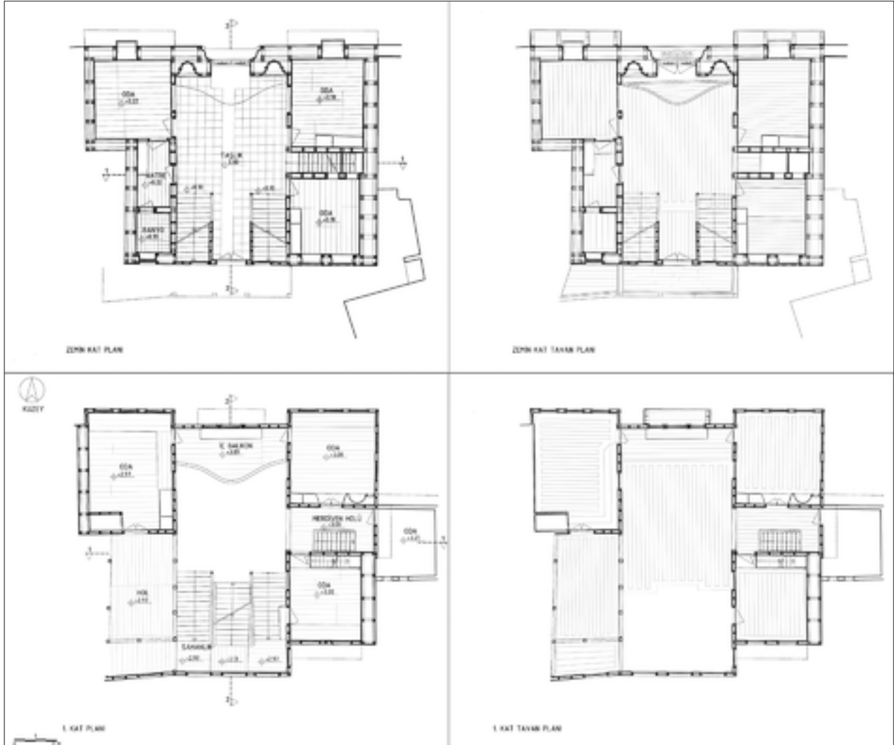
Şekil 12-1: Zemin, birinci ve ikinci katların döşeme ve tavan planları restitüsyon önerisi.
