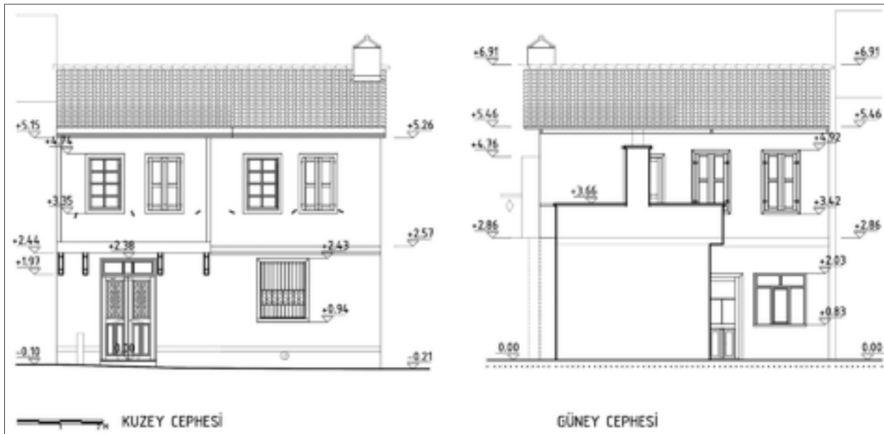
Şekil 10: Restorasyon kuzey ve güney cephesi önerileri.
