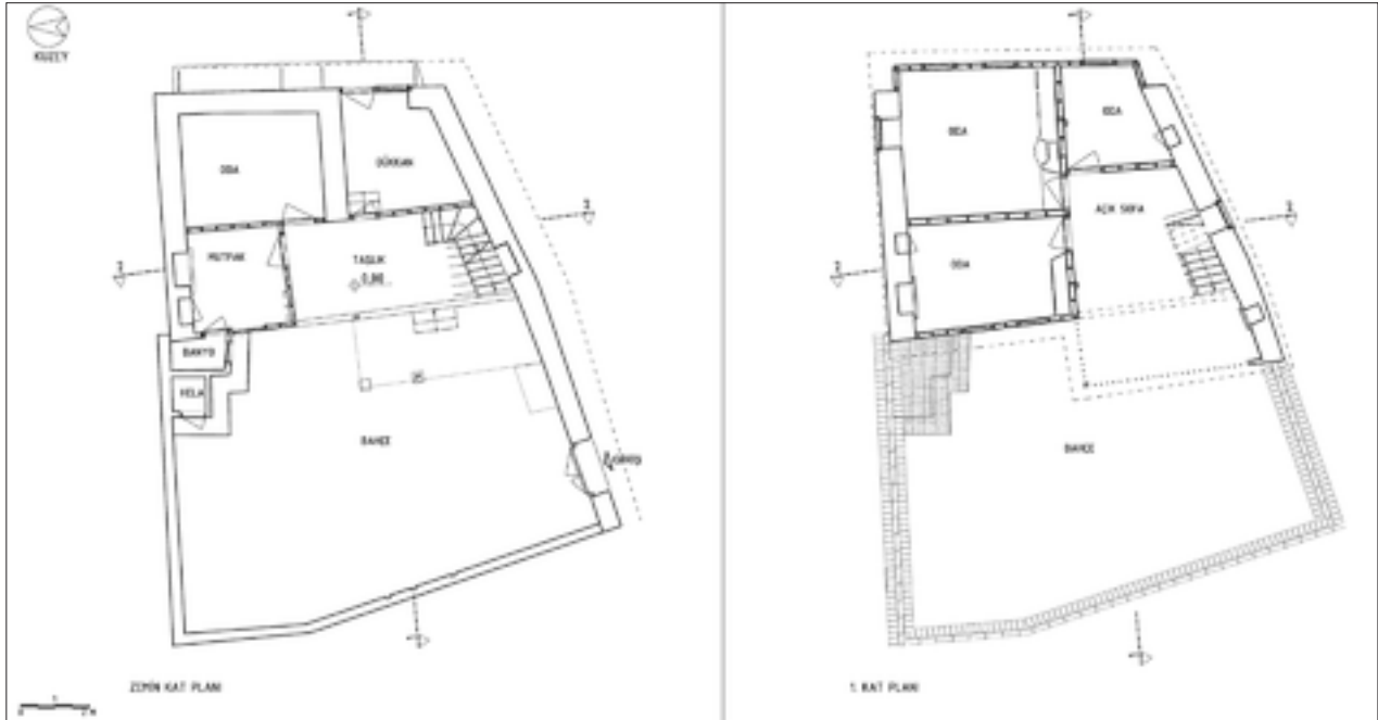
Şekil 9: Restitüsyon kat planları.
