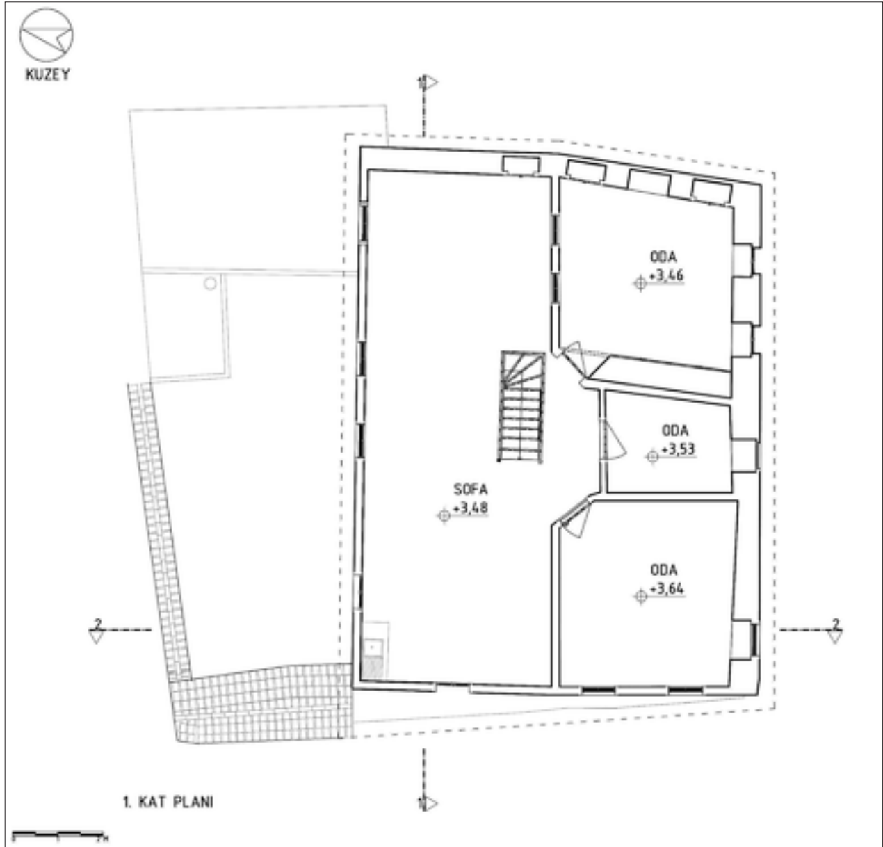
Şekil 4: Birinci kat planı rölövesi.
