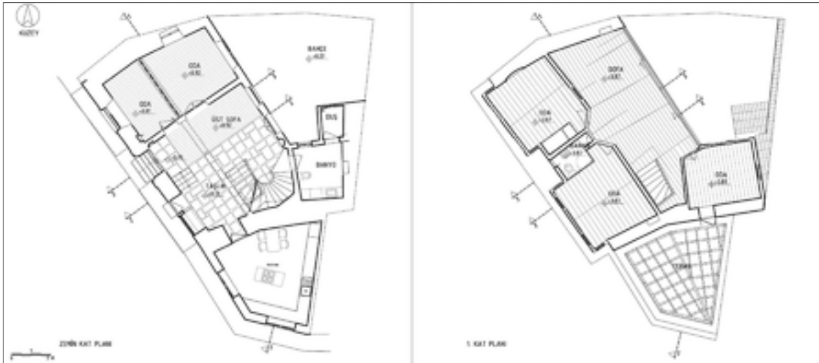
Şekil 14: Restorasyon tefrişli kat planları.
