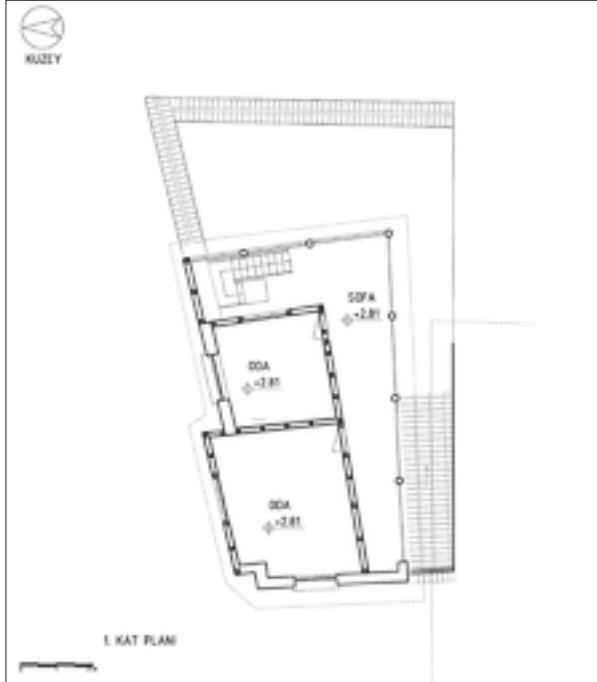
Şekil 14: Birinci kat planı restitüsyon önerisi.
