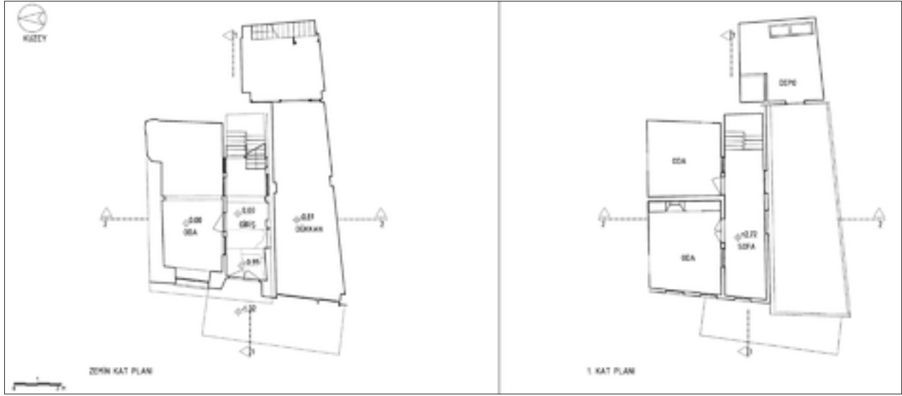
Şekil 4: Zemin ve birinci kat planı.
