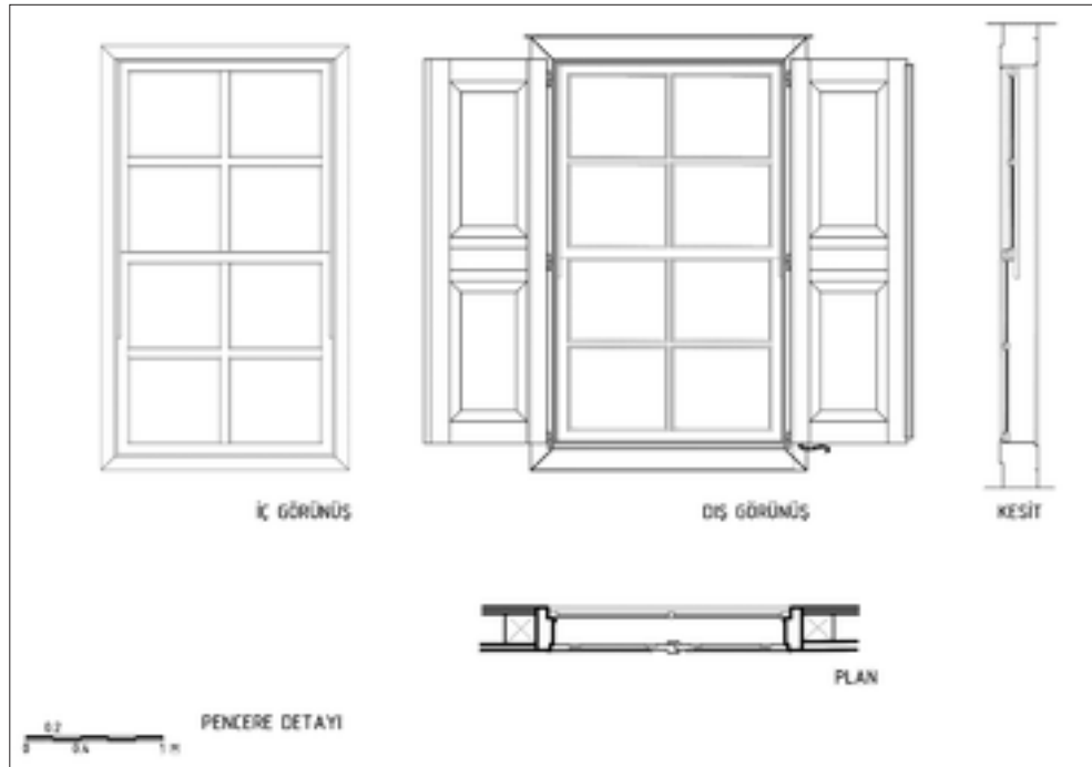
Şekil 15: Birinci dönem restitüsyon, giyotin pencere sistem detayı.
