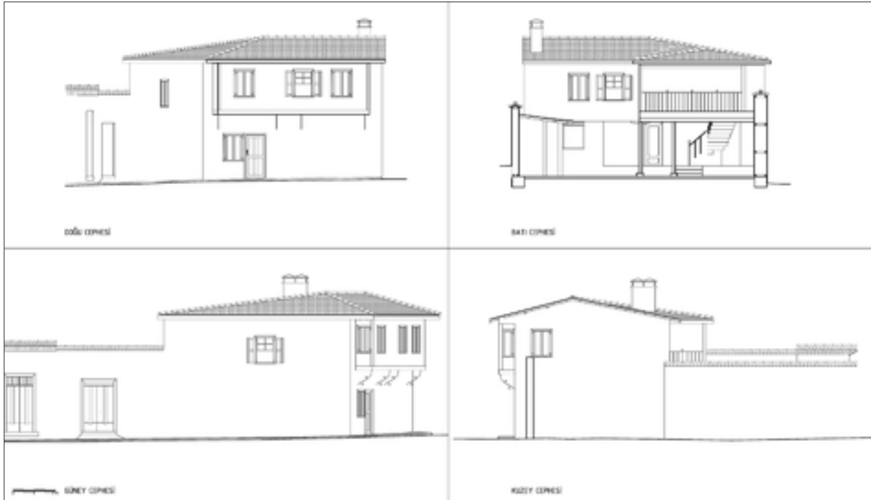
Şekil 11: Restitüsyon cepheler.
