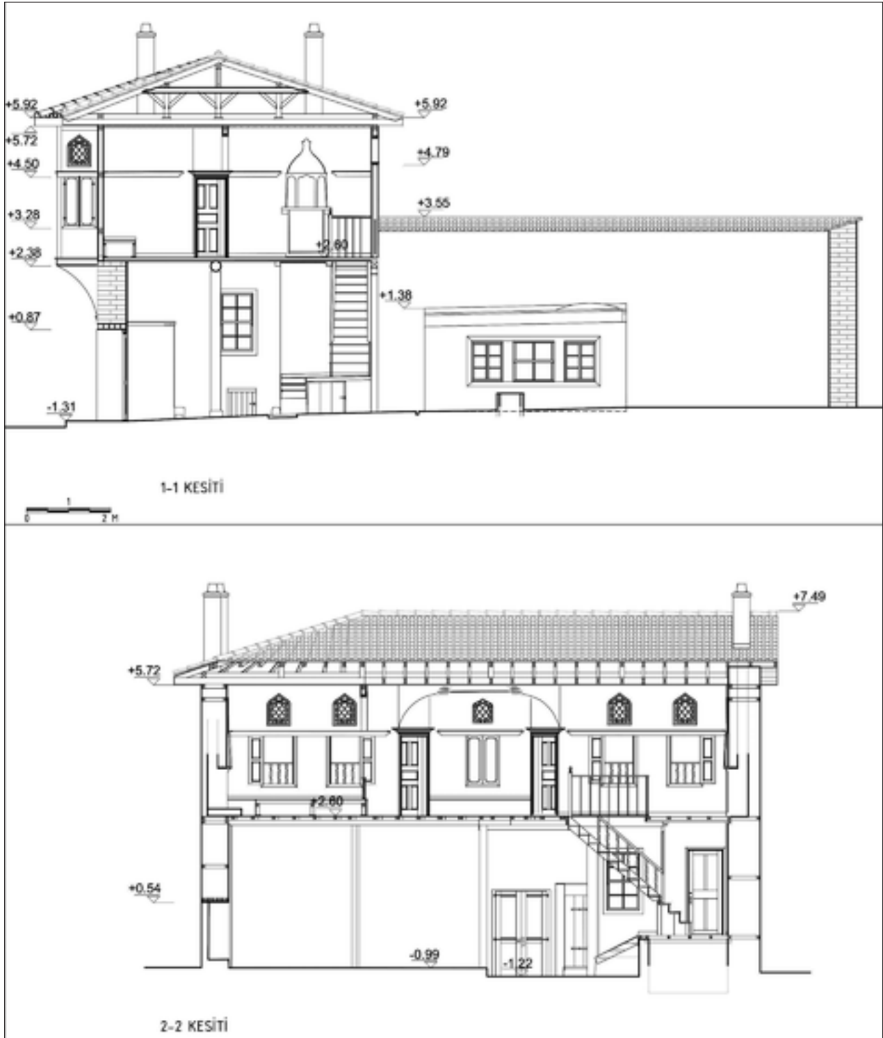
Şekil 20: 1. Dönem restitüsyonu kesitler.
