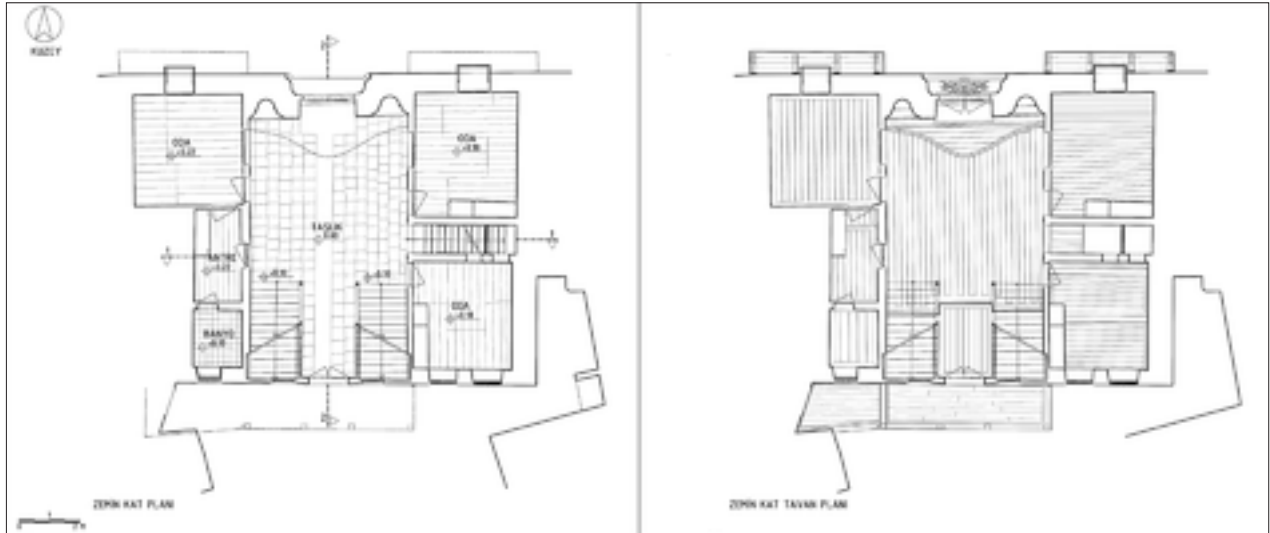
Şekil 3: Zemin kat Döşeme ve tavan planları.
