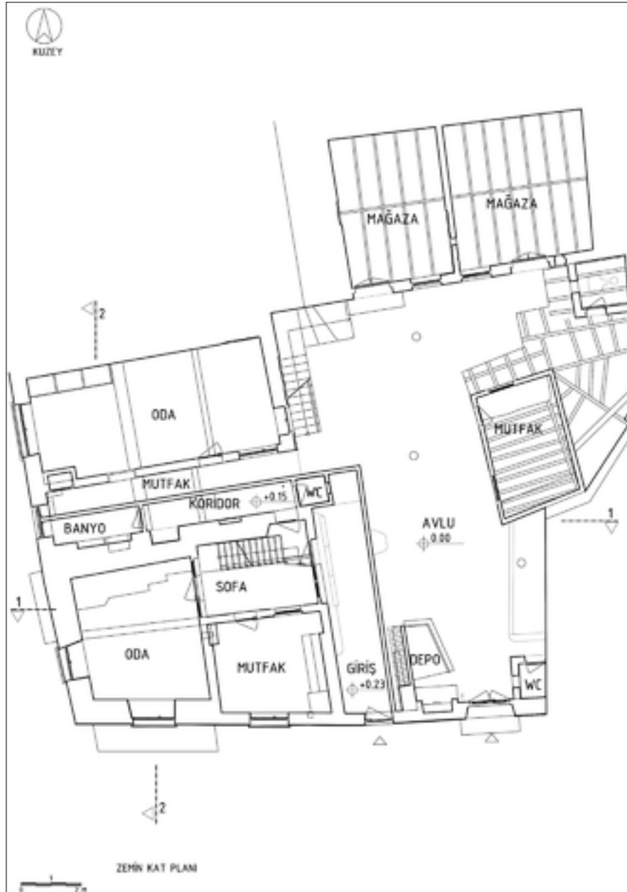
Şekil 3: Zemin kat döşeme planı.
