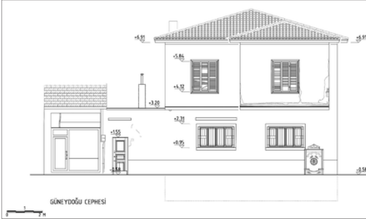
Şekil 12: Güneydoğu (Cumhuriyet Caddesi) cephesi rölövesi.
