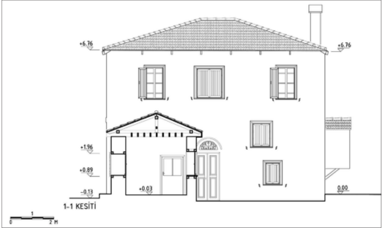
Şekil 15: Restitüsyon, 1-1 kesiti.
