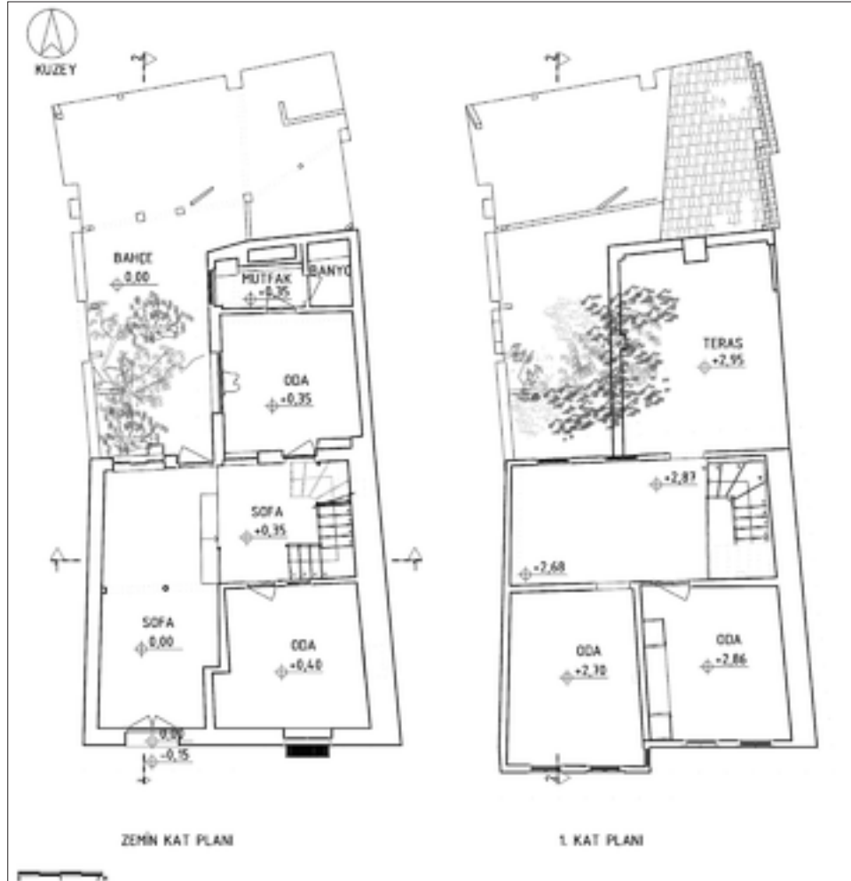
Şekil 2: Rölöve zemin ve 1. kat planı.
