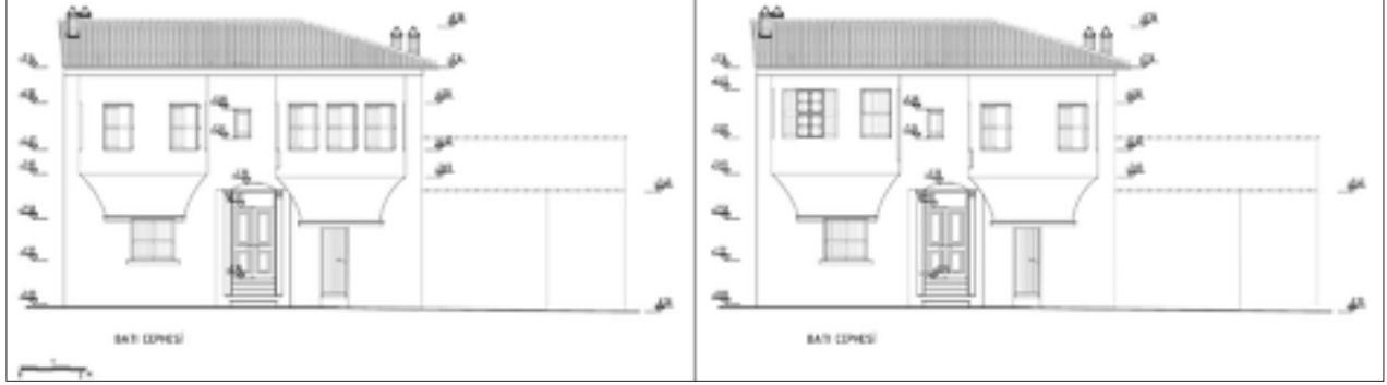
Şekil 12: 1. ve 2. dönem restitüsyon ön cephe görünüşleri.
