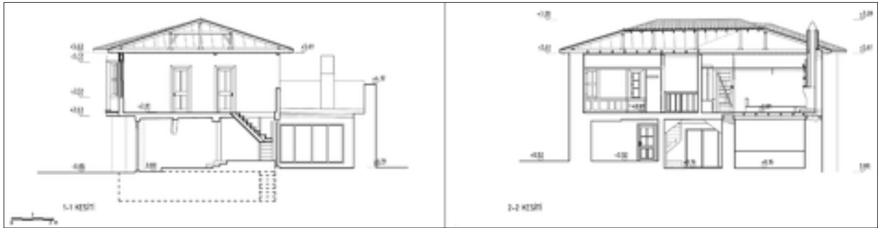
Şekil 19: Restorasyon kesitler.
