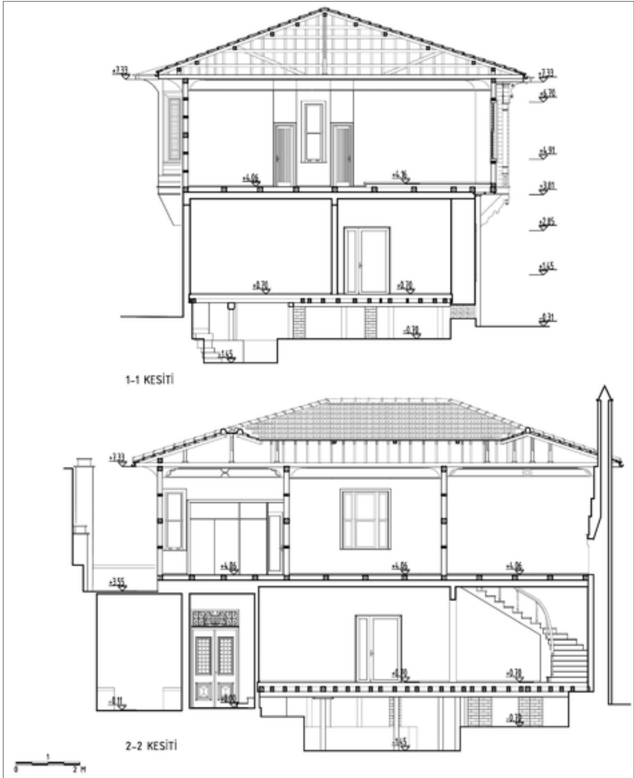
Şekil 11: Birinci dönem restitüsyon enine ve boyuna kesit.
