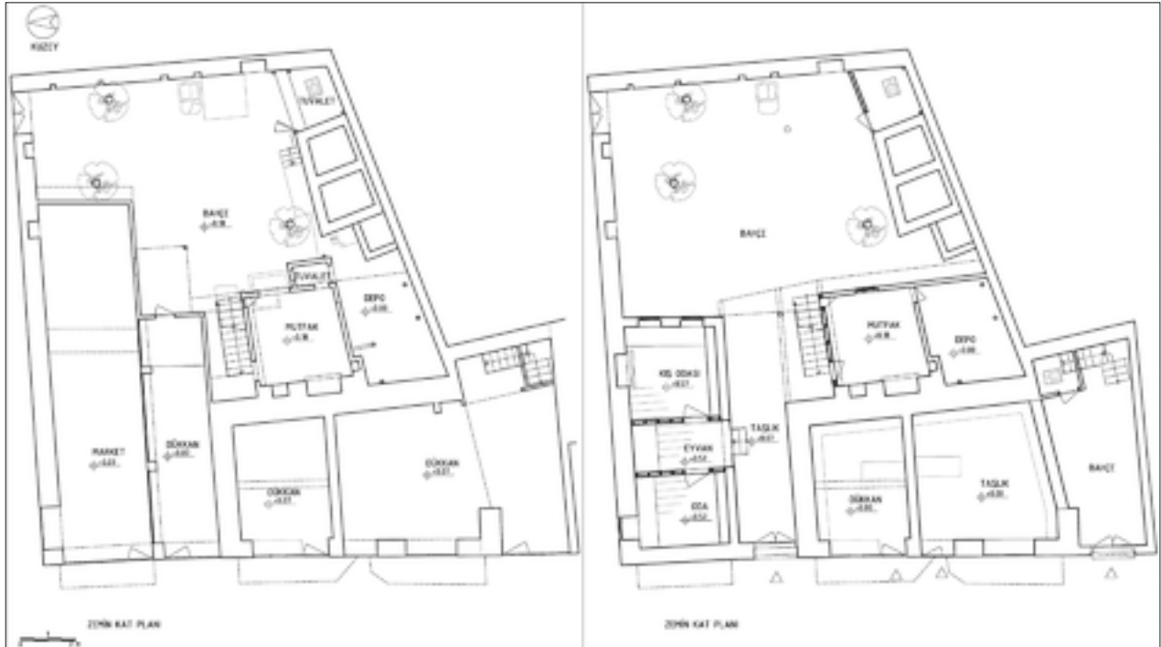
Şekil 17: Alt kat rölövesi (solda) ve ikinci dönem restitüsyonu (sağda).
