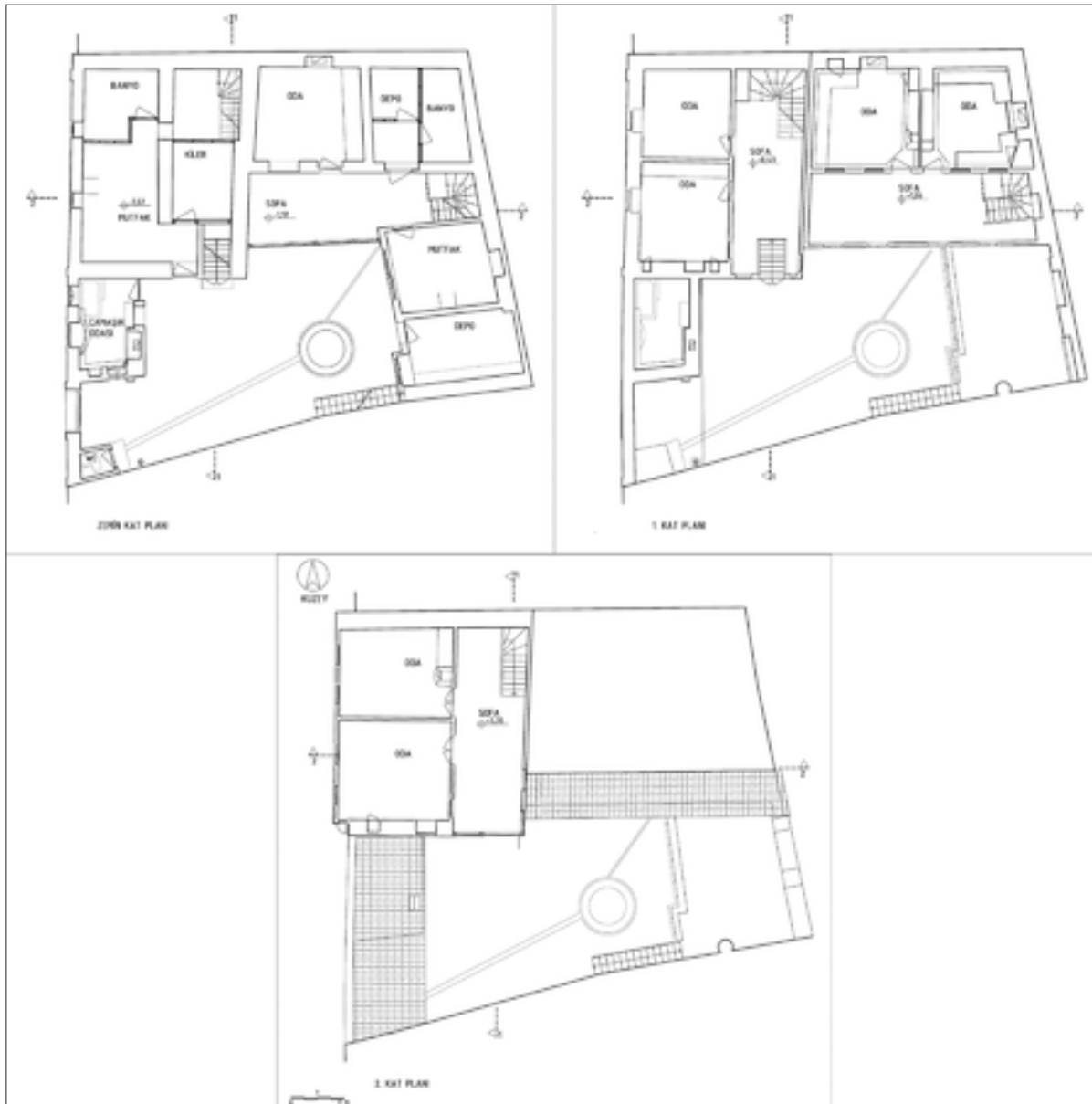
Şekil 14: Restorasyon kat planları.
