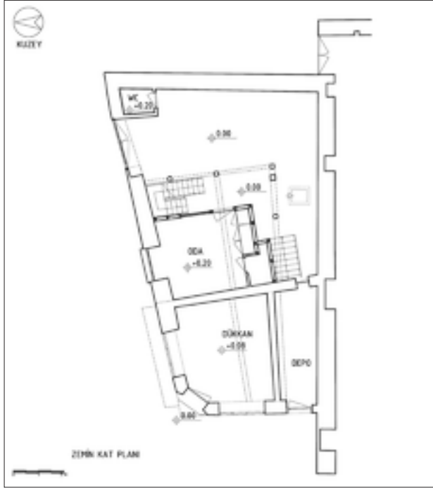
Şekil 11: Zemin kat planı restitüsyon önerisi.
