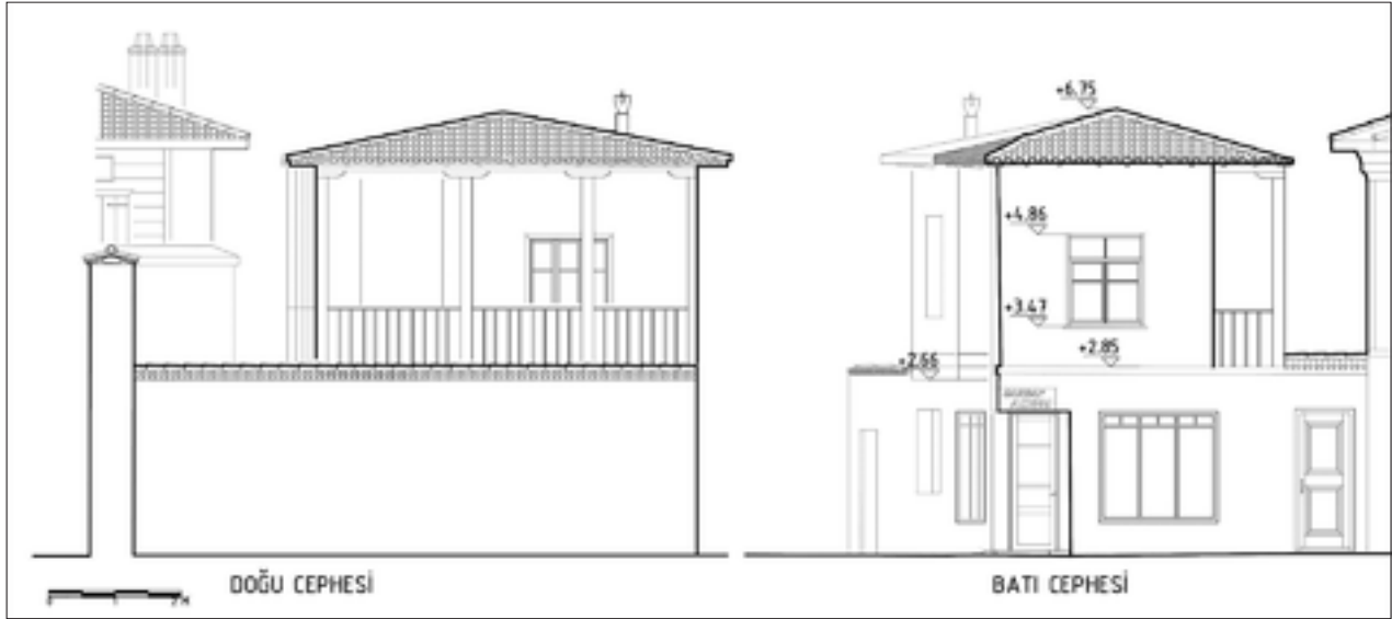
Şekil 17: Batı ve doğu cephesi restitüsyon önerisi.
