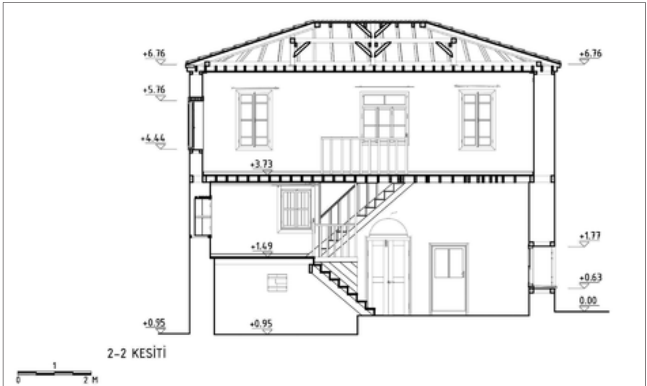
Şekil 16: Restitüsyon, 2-2 kesiti.
