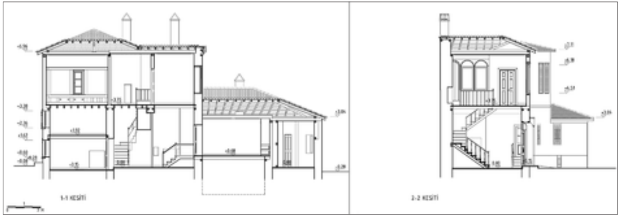
Şekil 15: Restorasyon enine ve boyuna kesit.
