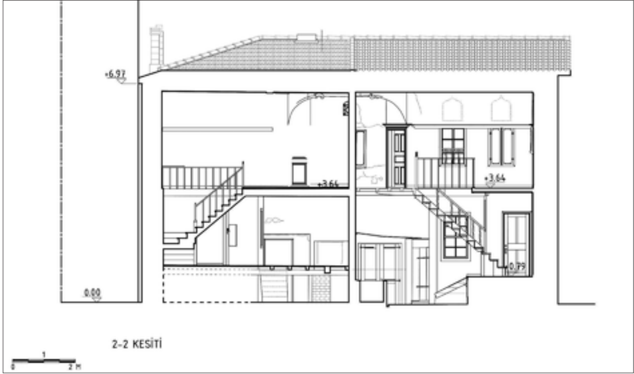
Şekil 16: Enine kesit rölövesi.
