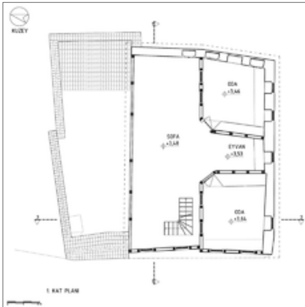
Şekil 13: Birinci kat planı restitüsyon önerisi.
