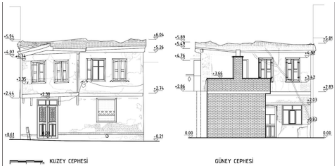
Şekil 3: Rölöve kuzey ve güney cephesi.
