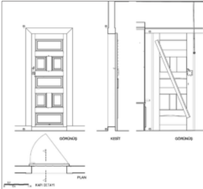
Şekil 10: Özgün iç kapı detayı.
