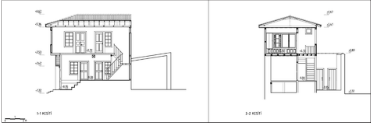
Şekil 16: 1-1 Kesiti ve 2-2 kesiti.
