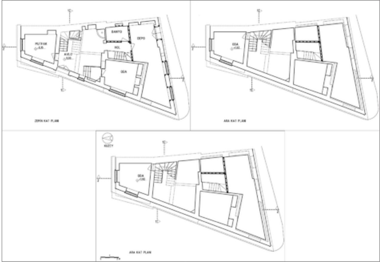
Şekil 14: Restorasyon kat planları.
