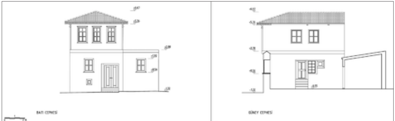
Şekil 20: Ön ve güney cephe için ikinci dönem restitüsyon önerileri.
