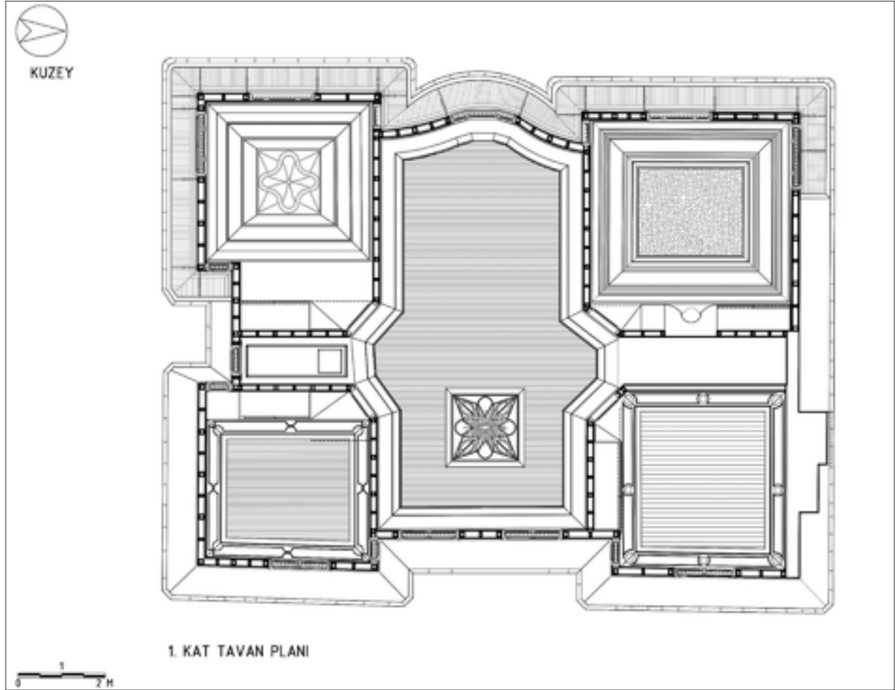
Şekil 10: Birinci dönem restitüsyon tavan planı.
