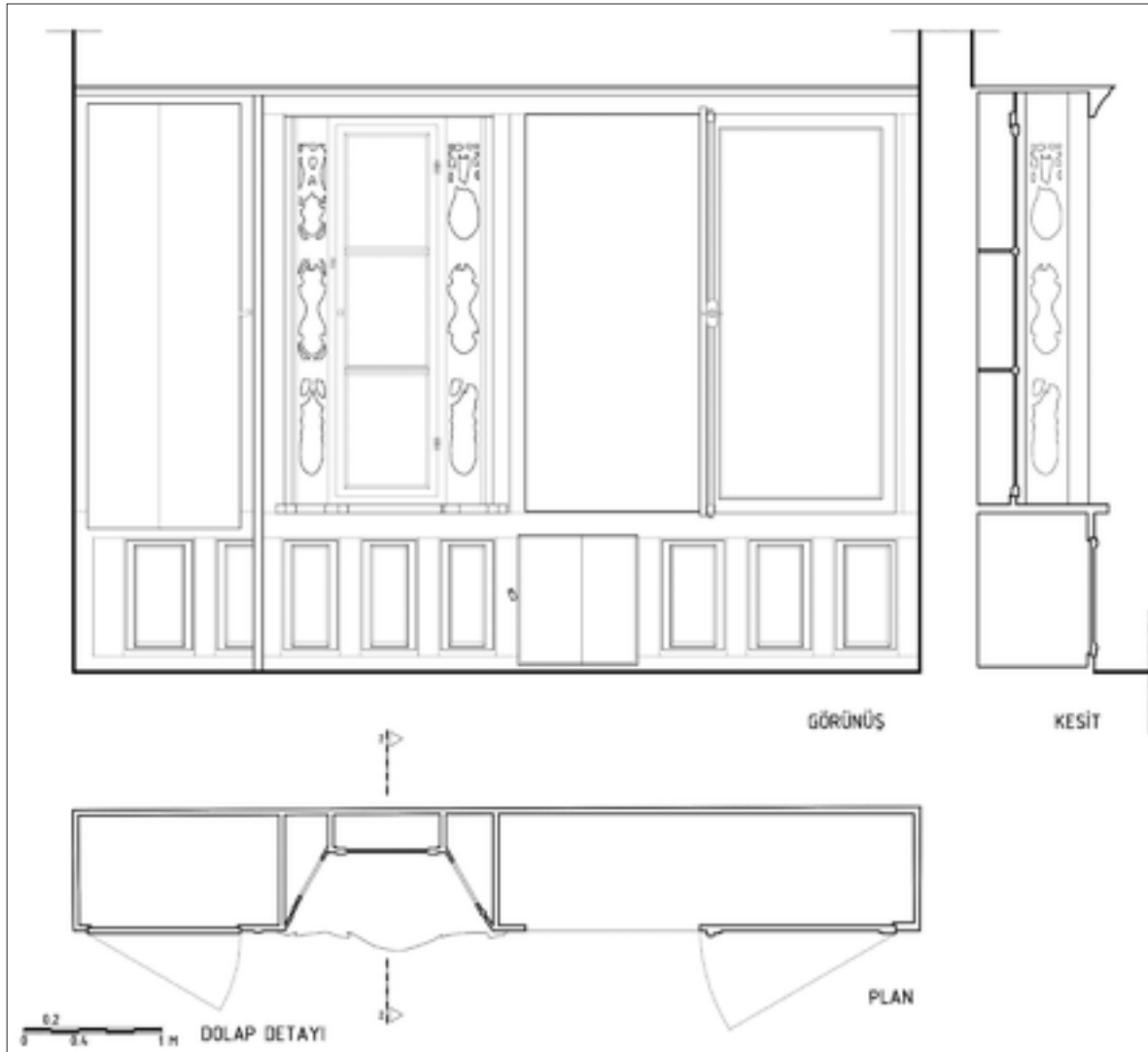
Şekil 13: Birinci katta bulunan dolap detayı.
