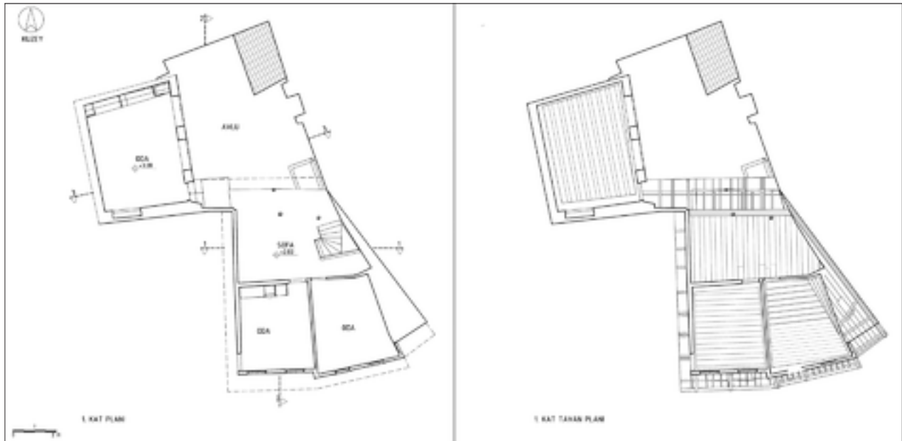
Şekil 7: Rölöve 1. kat döşeme ve tavan planı.
