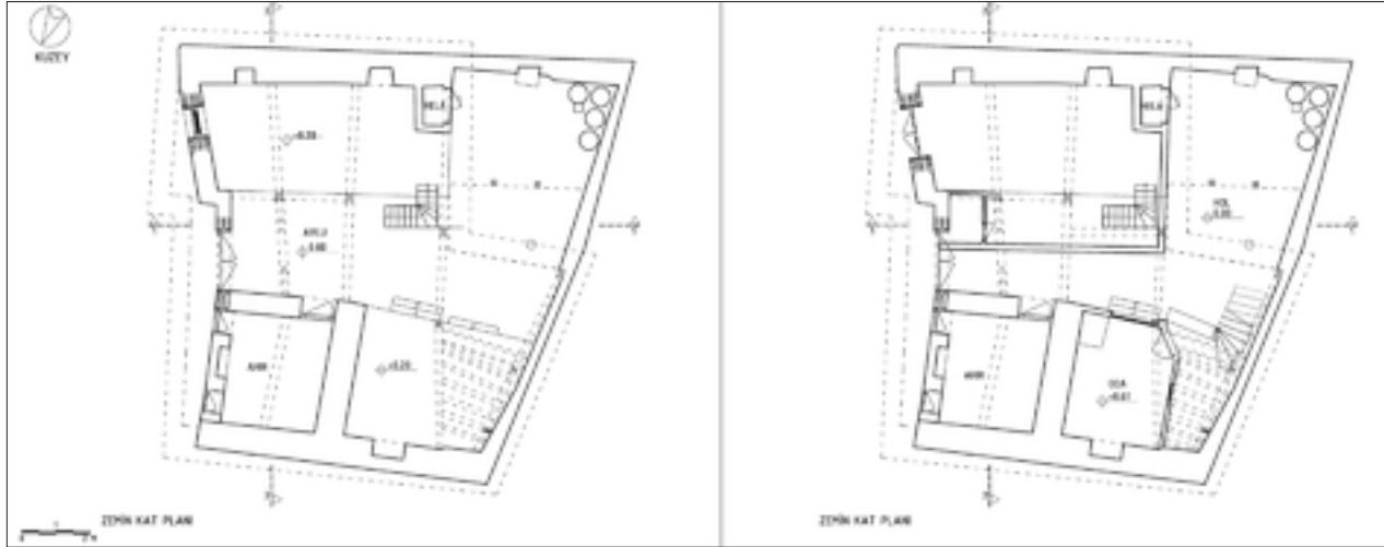
Şekil 14: 1. dönem ve 2. dönem restitüsyon önerisi zemin kat planı.
