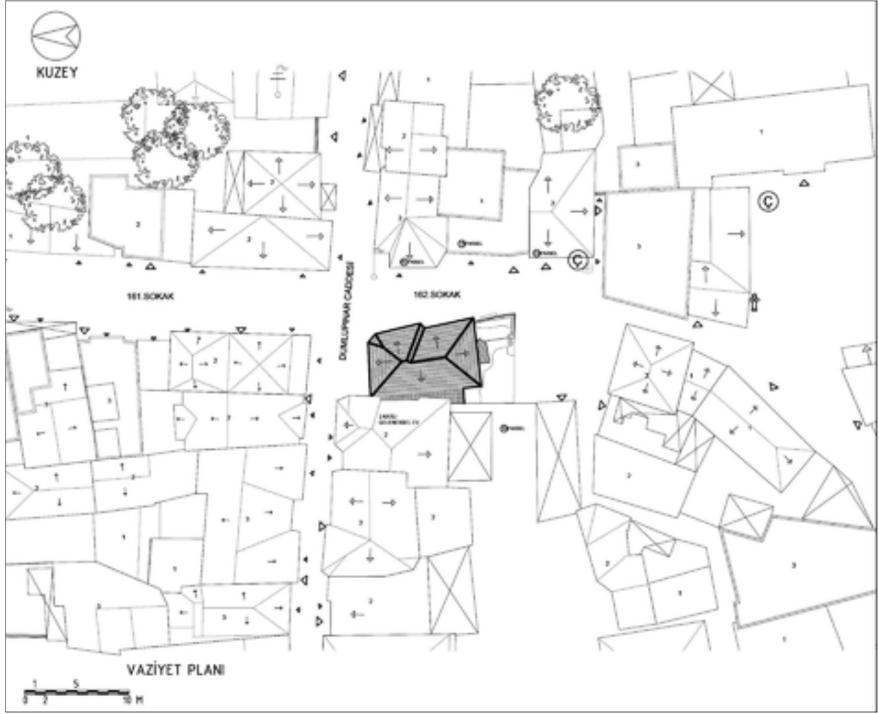
Şekil 3: Vaziyet planı rölovesi.
