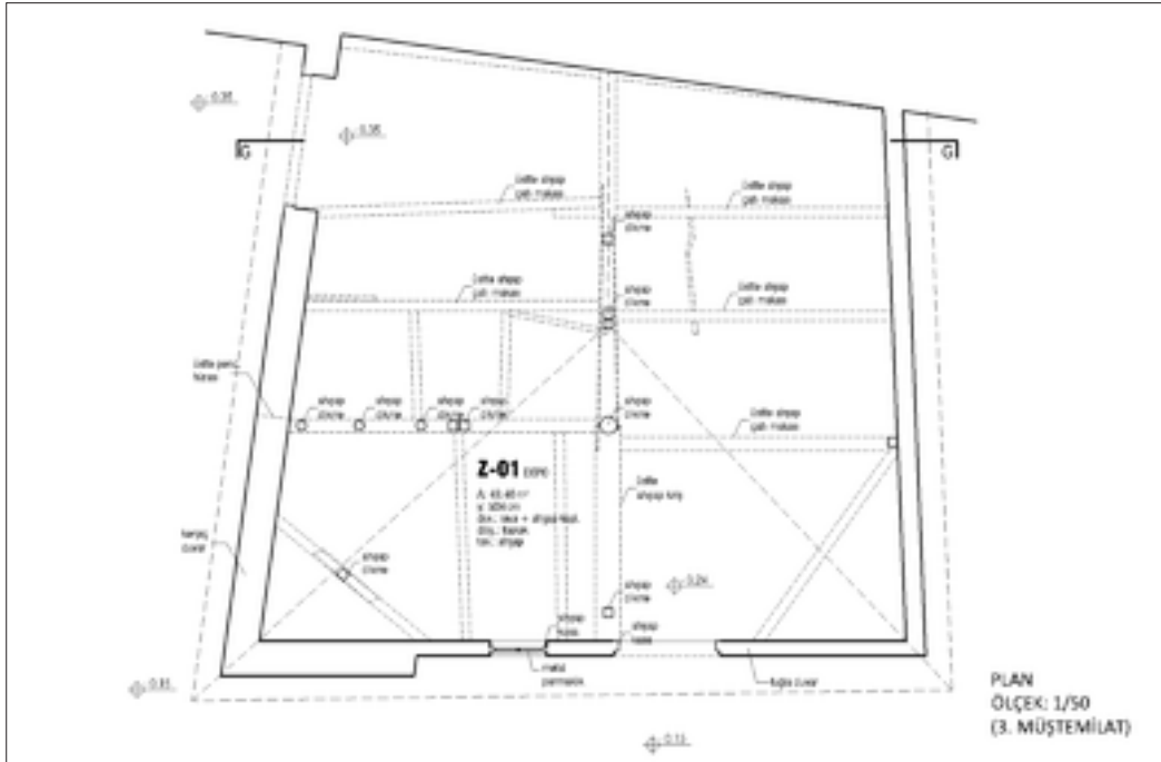
Şekil 23: Üçüncü müştemilat planı (rölöve).
