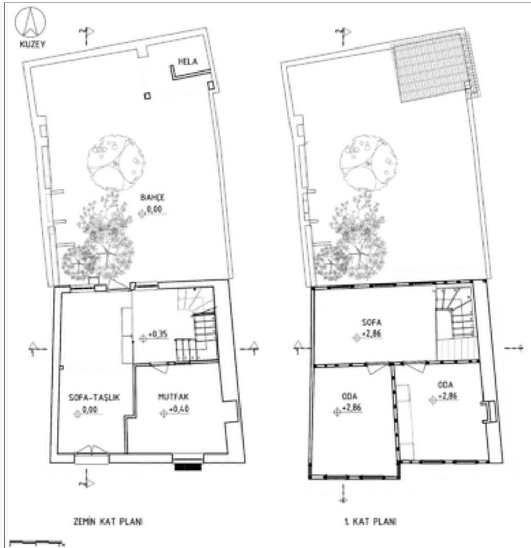
Şekil 5: Restitüsyon (1. Dönem) zemin ve 1. kat planı.
