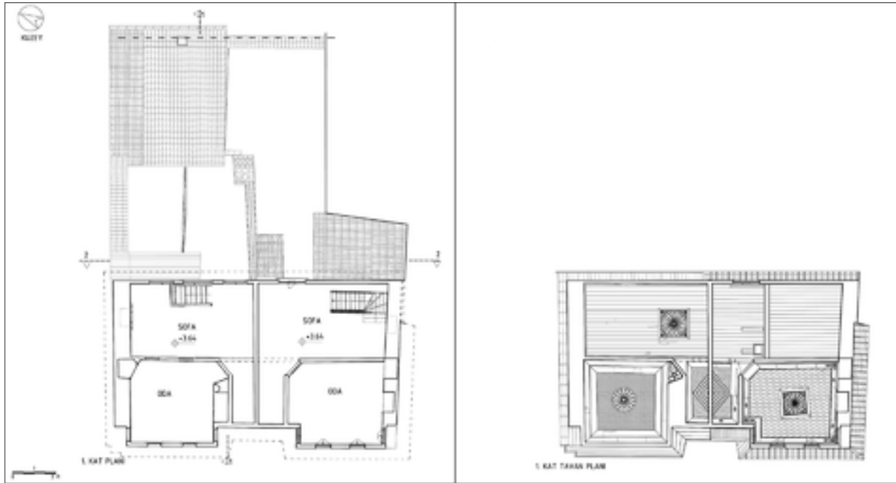
Şekil 6: Birinci kat döşeme planı ve tavan planı rölevelleri.
