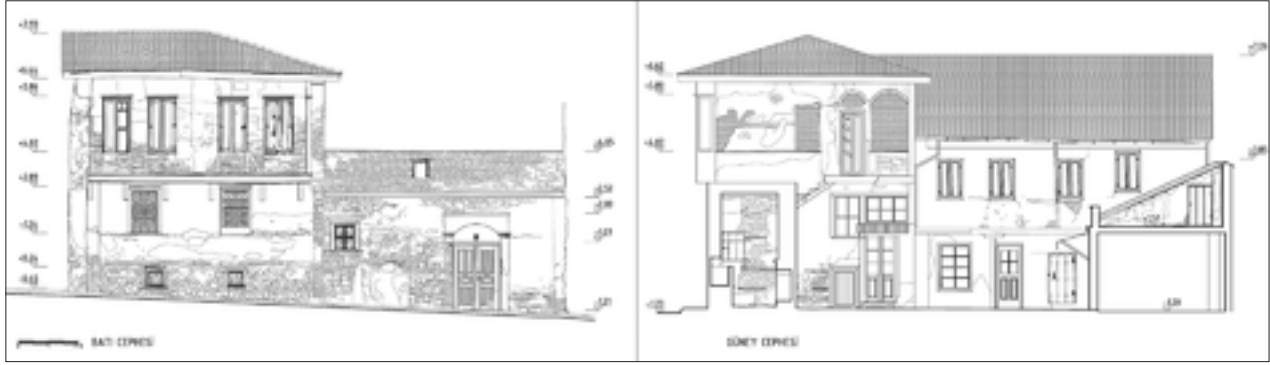
Şekil 10: Rölöve cepheler.
