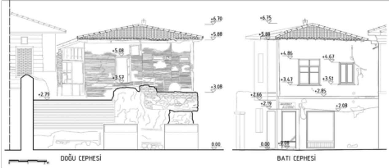
Şekil 8: Doğu ve kuzey cephesi rölöveleri.
