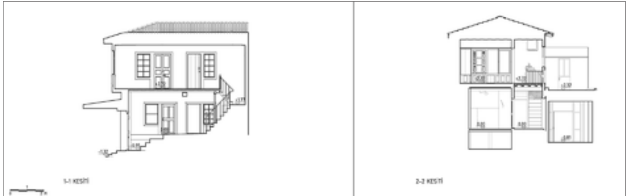
Şekil 5: Kesit 1 ve kesit 2.
