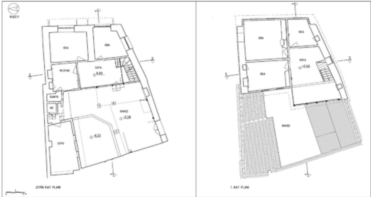
Şekil 6: Rolöve kat planları.
