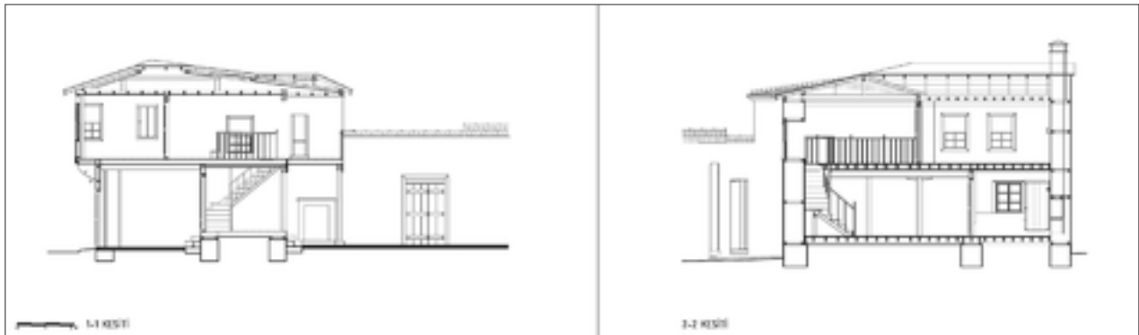
Şekil 10: Restitüsyon enine ve boyuna kesit.
