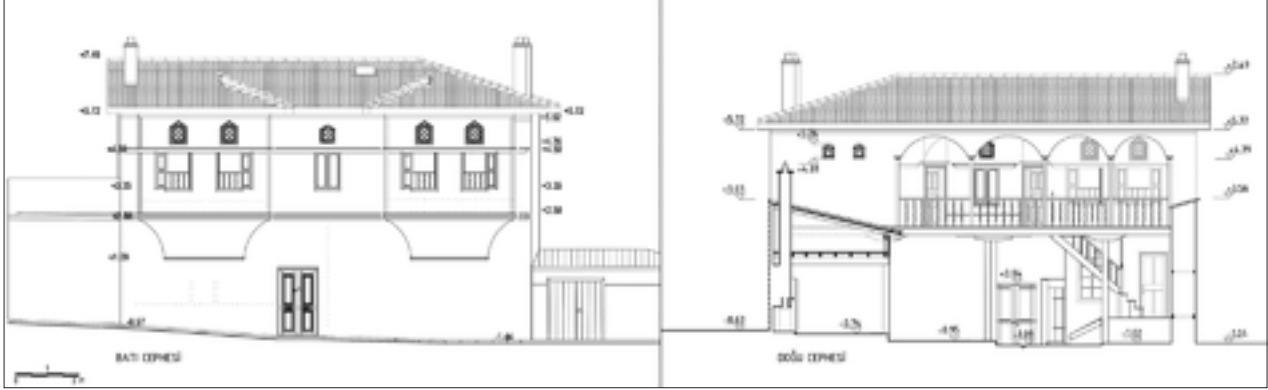
Şekil 21: 1. Dönem restitüsyonu sokak ve avlu cepheleri.
