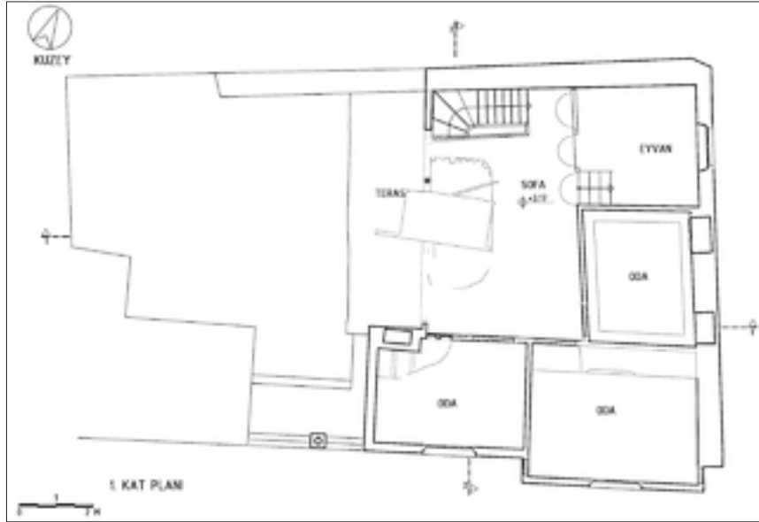
Şekil 11: Birinci kat plan rölovesi.
