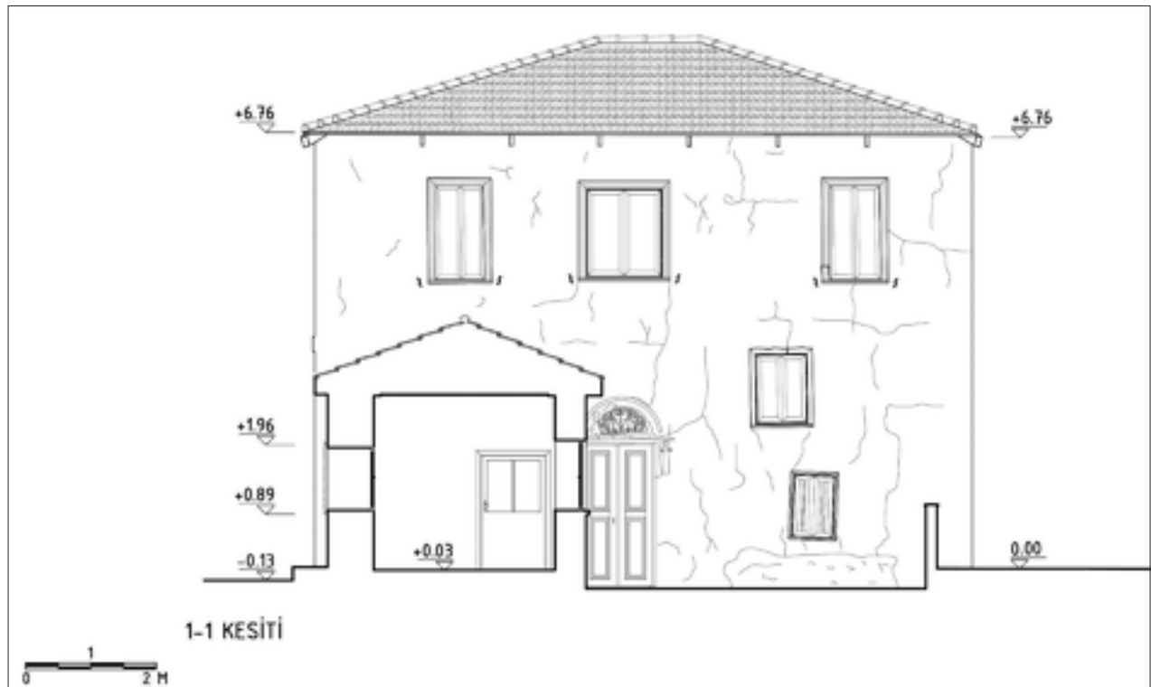
Şekil 8: Rölöve, 1-1 kesiti.
