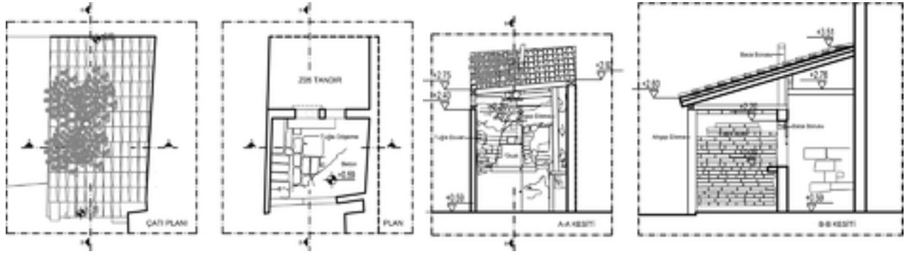
Şekil 4: Tandır, plan, kesit, görünüş.
