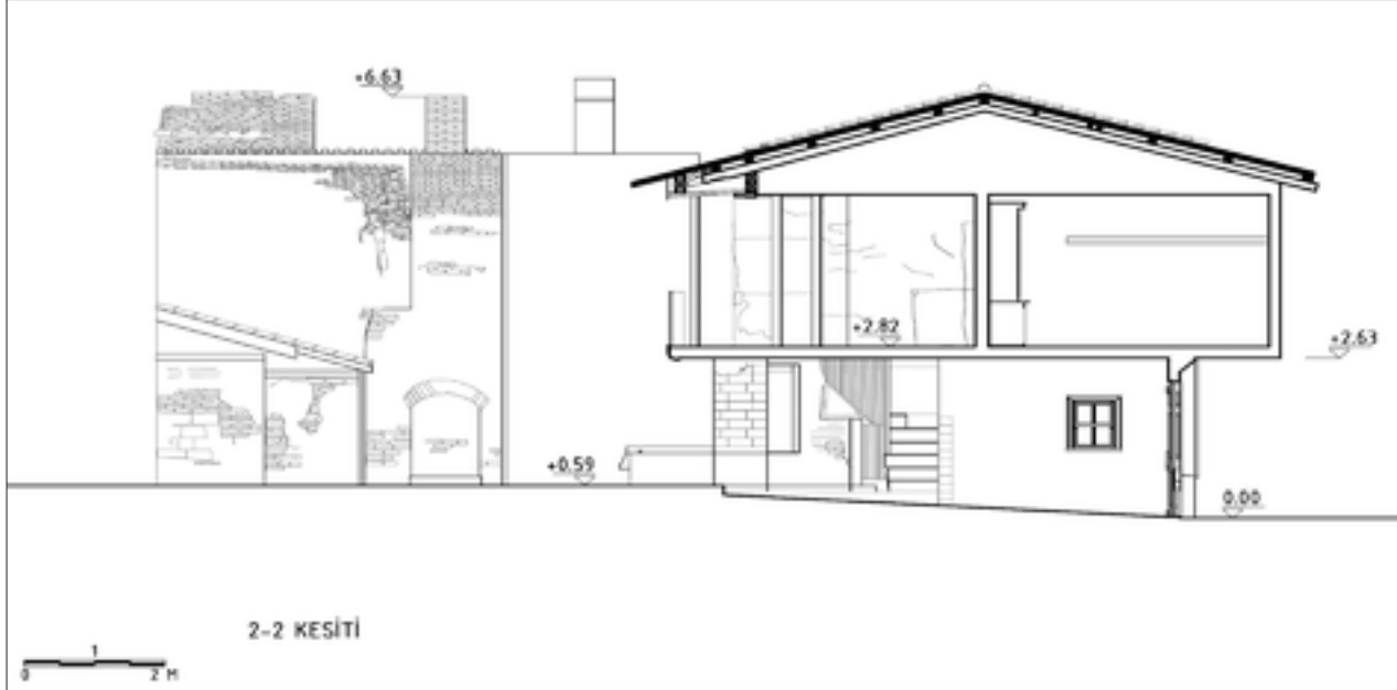
Şekil 11: Rölöve A-A kesit.
