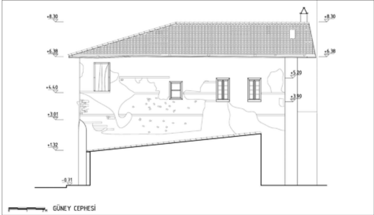
Şekil 7: Güneydoğu cephesi rölövesi.
