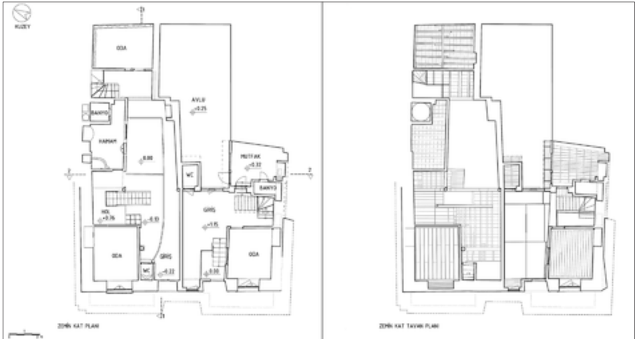
Şekil 5: Zemin kat döşeme planı ve tavan planı rölöveleri.
