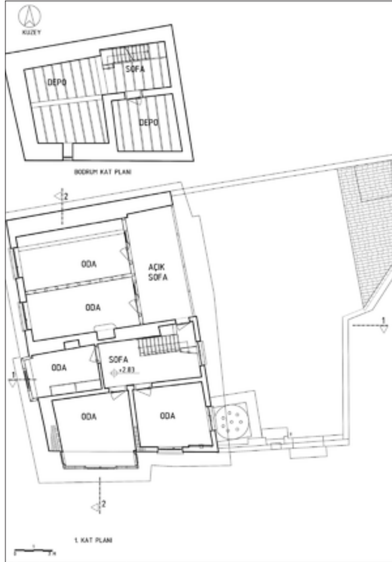
Şekil 10: Bodrum ve birinci kat döşeme planları.
