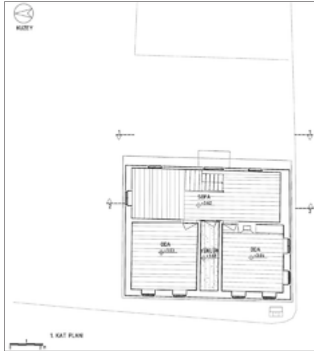
Şekil 7: Rölöve kat planları - birinci kat planı.
