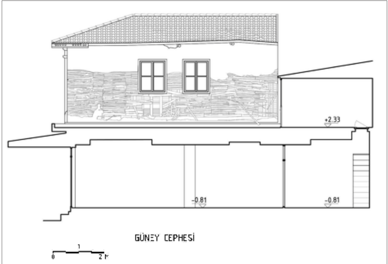
Şekil 11: Güney cephesi.
