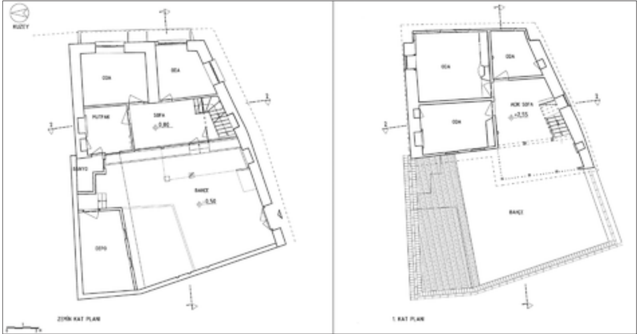
Şekil 12: Restorasyon kat planları.
