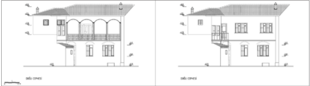
Şekil 13: 1. ve 2. dönem restitüsyon arka cephe görünüşleri.
