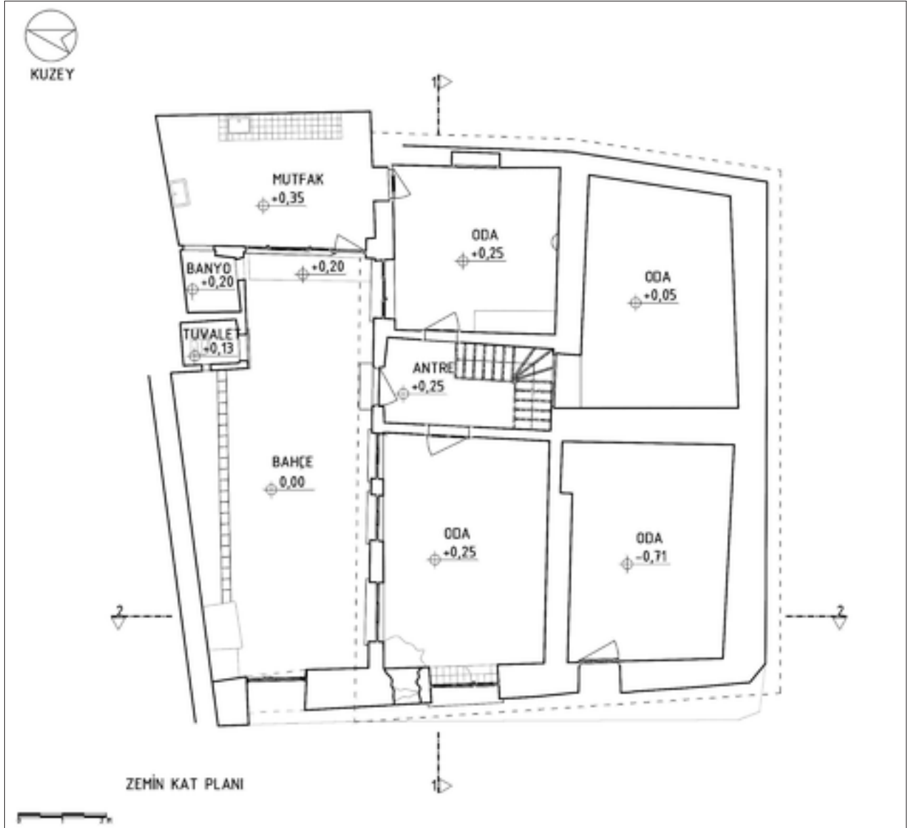
Şekil 3: Zemin kat planı rölövesi.
