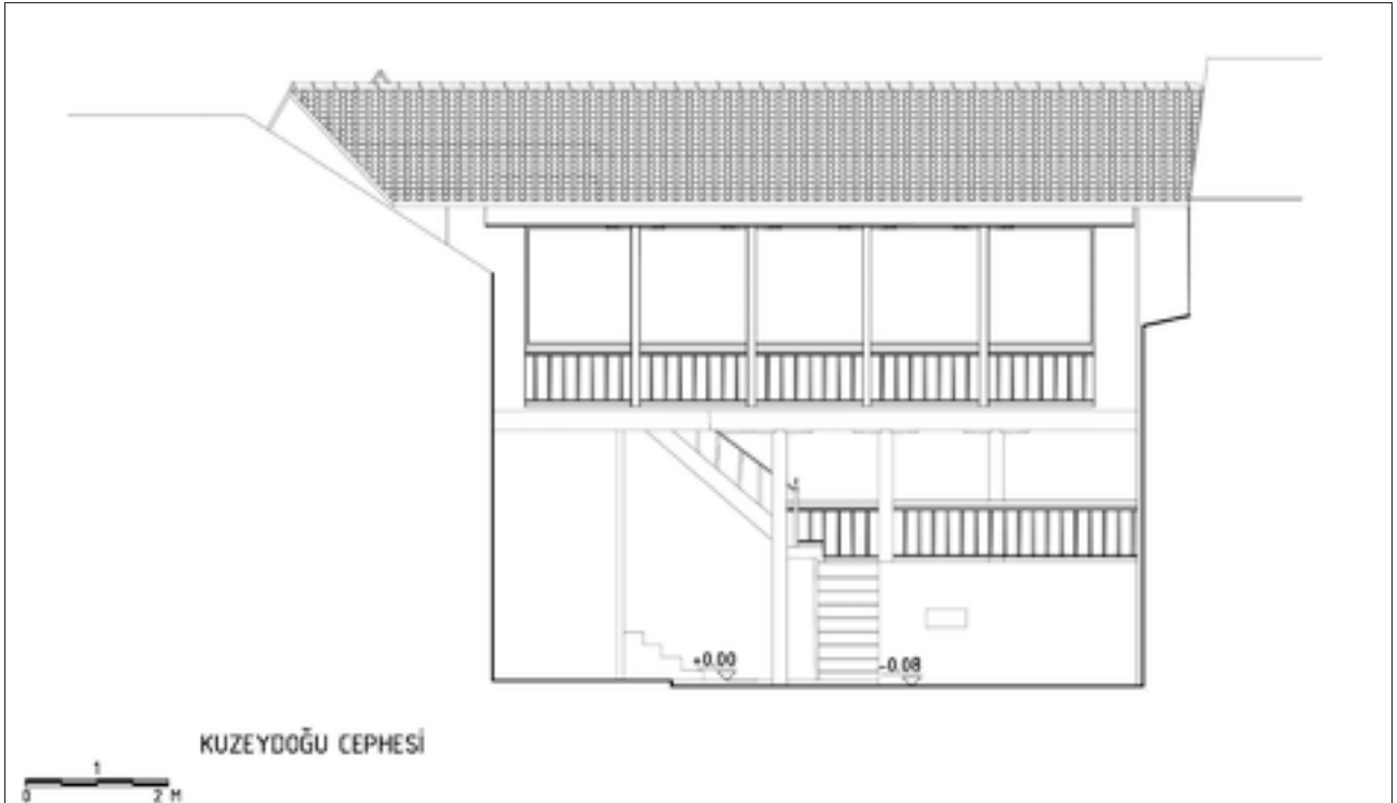
Şekil 21: 2-2 kesiti (kuzeydoğu cephesi).
