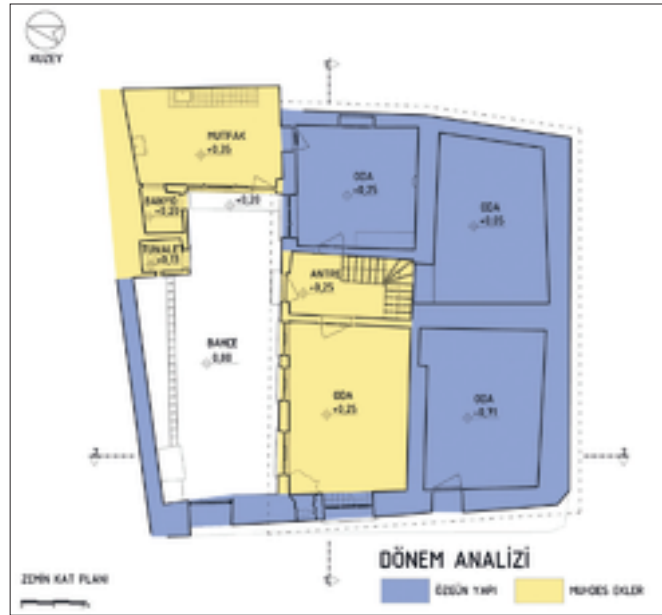
Şekil 9: Zemin kat dönem analizi.
