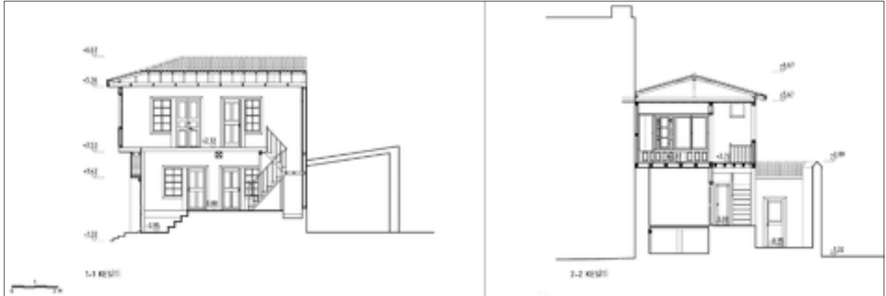
Şekil 22: 1-1 Kesiti ve 2-2 kesiti.
