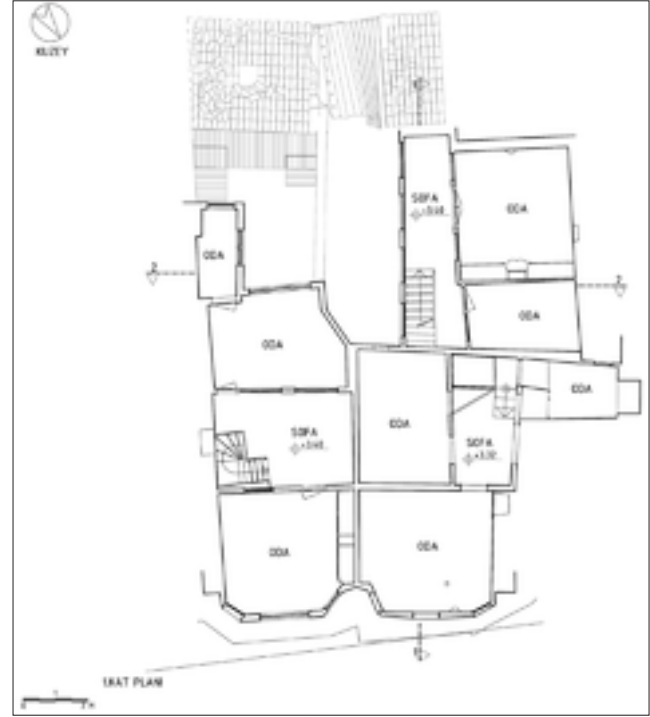
Şekil 4: Rölöve 1. kat planı.
