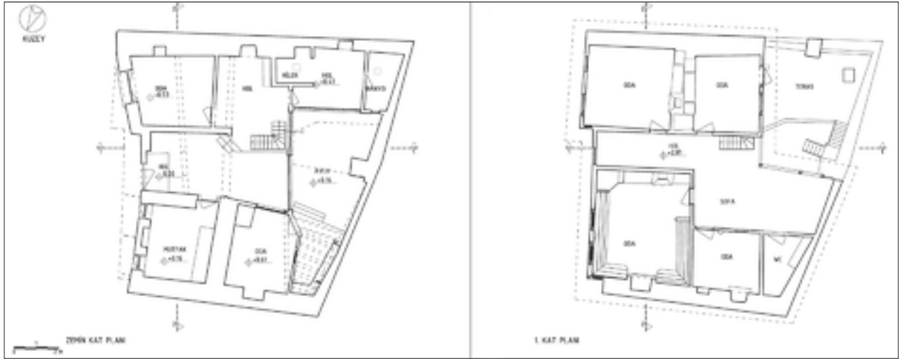
Şekil 18: Restorasyon müdahaleleri zemin ve 1. kat planı.
