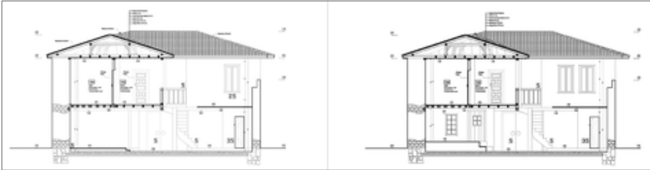
Şekil 17: Arka Cephinin 1. Dönem ve 2. Dönem Restitüsyon Önerisi
