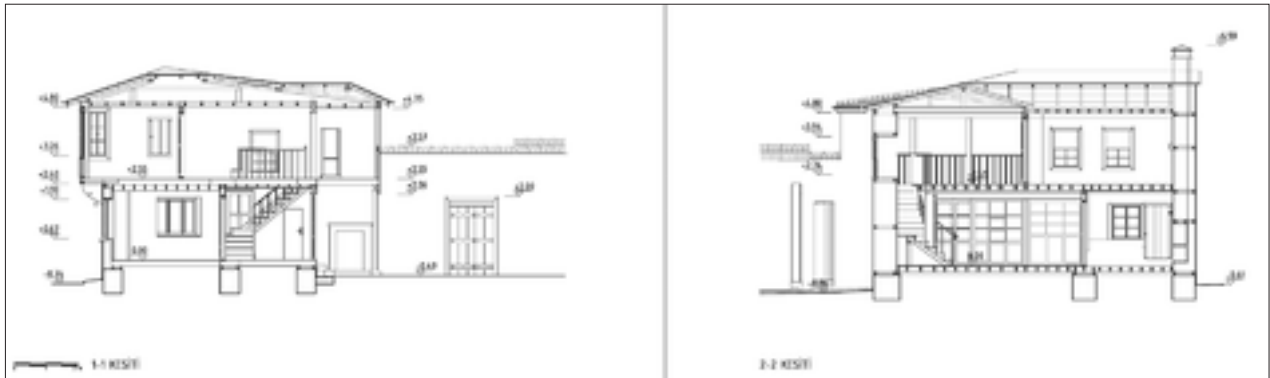
Şekil 13: Restorasyon enine ve boyuna kesit.
