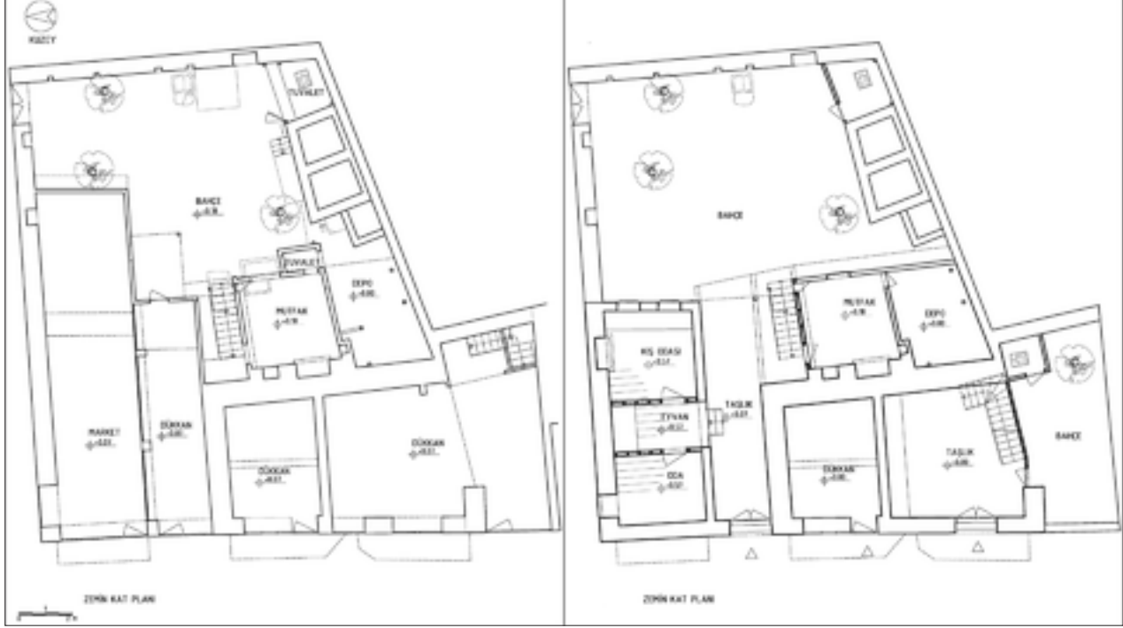
Şekil 6: Alt kat rölovesi (solda) ve birinci dönem restitüsyonu (sağda).
