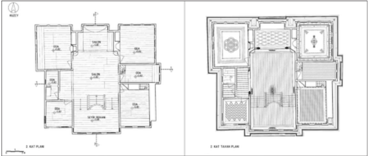
Şekil 6: İkinci kat döşeme ve tavan planları.
