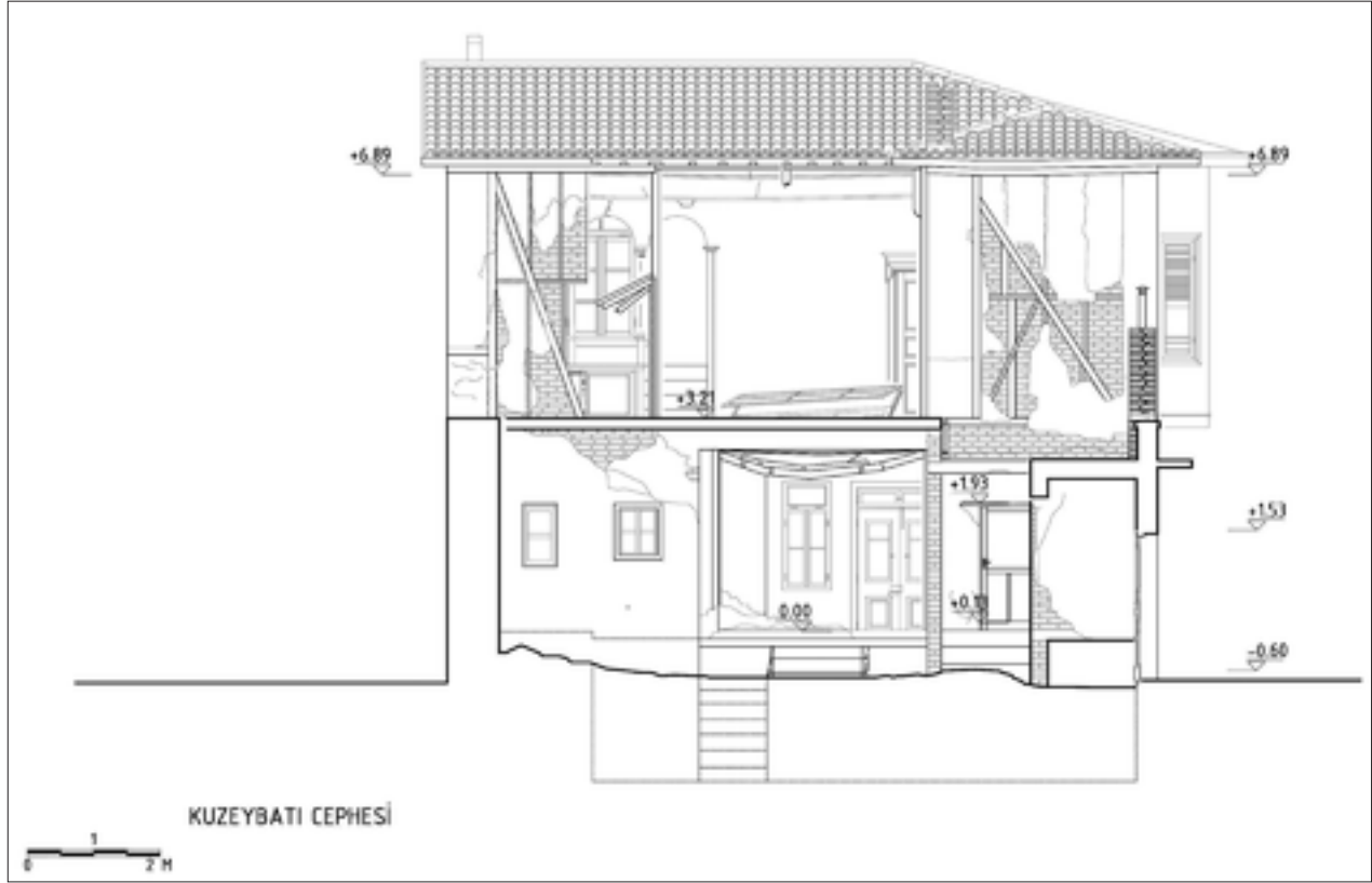
Şekil 14: Kuzeybatı (Avlu) cephesi rölövesi.
