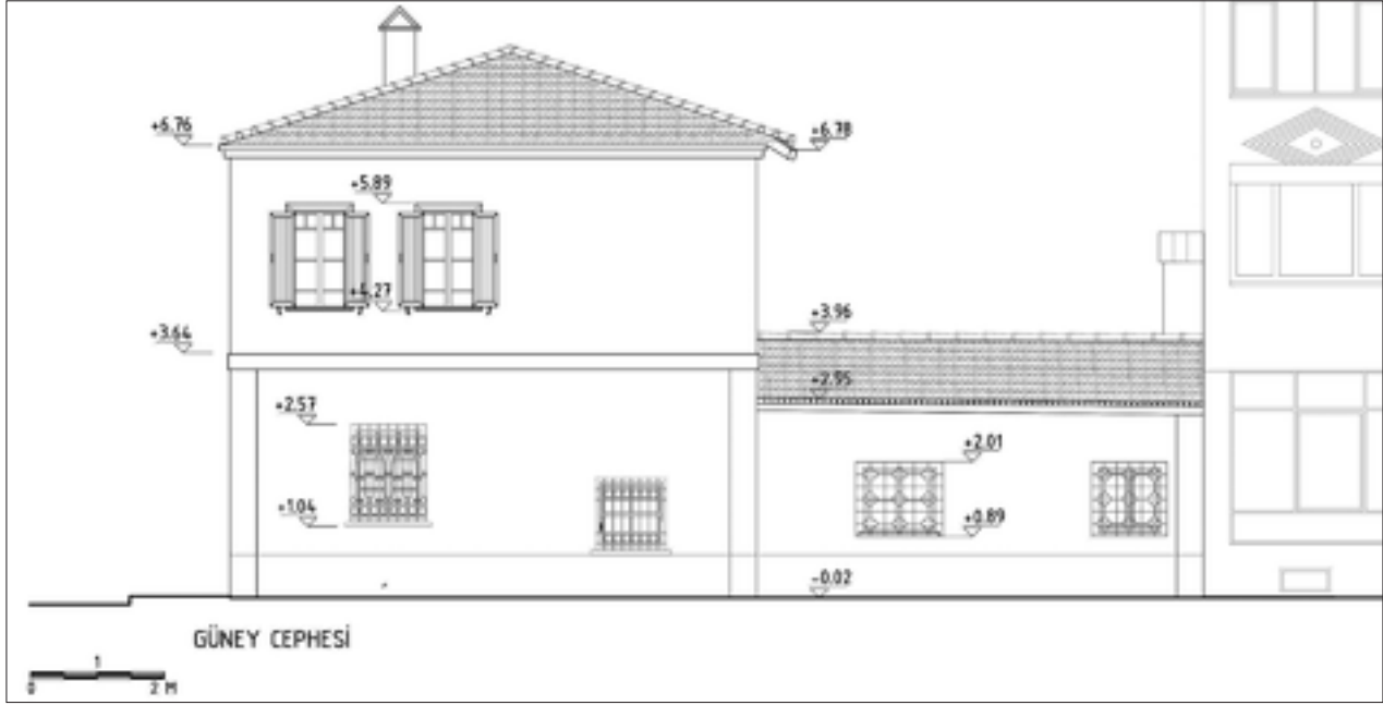
Şekil 25: Restorasyon, yan cephe - Muhlis Kayalı Cad. görünüşü.
