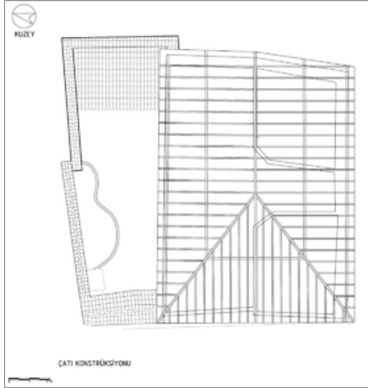
Şekil 20: Çatı konstrüksiyonu restorasyon önerisi.
