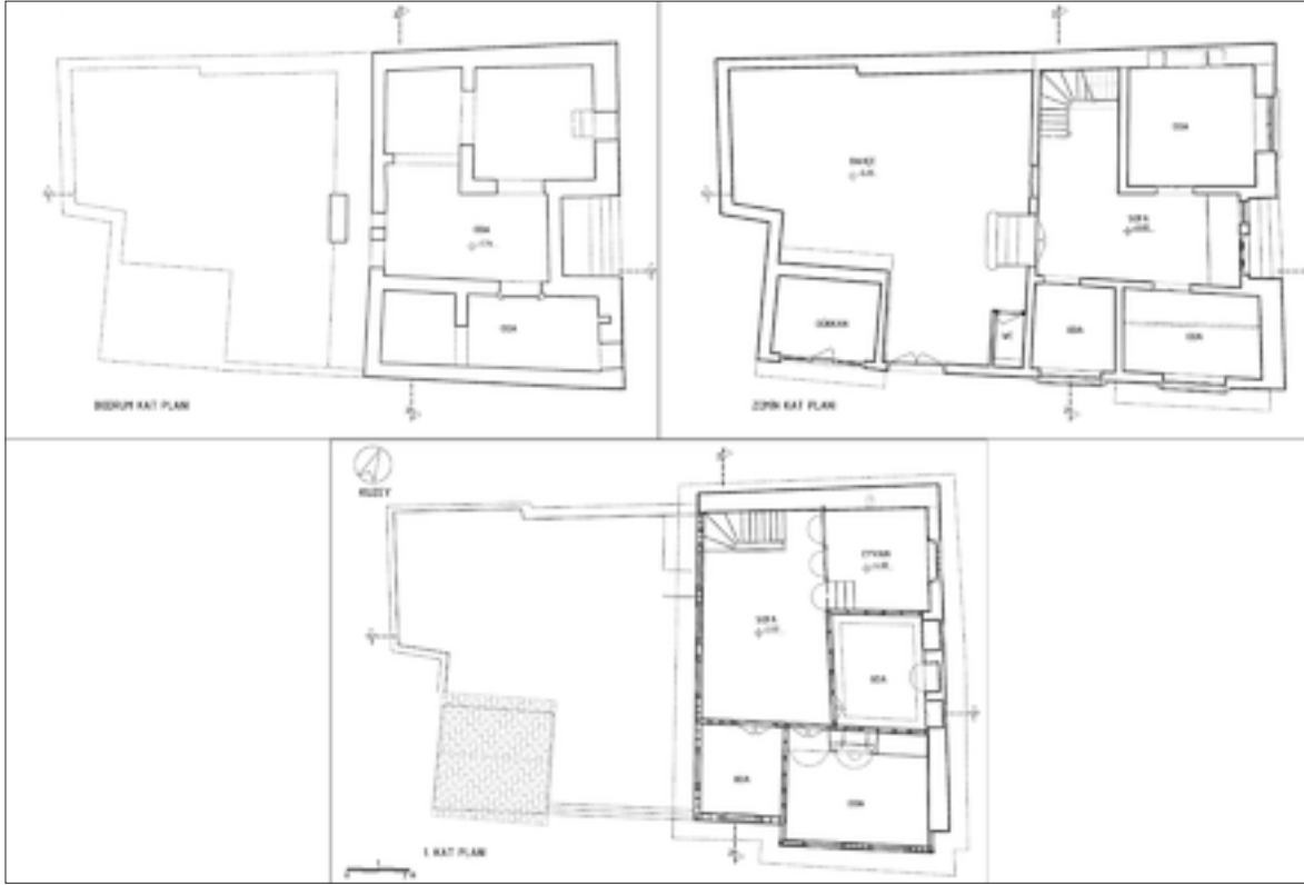
Şekil 18: I. Dönem restitüsyon kat planları.
