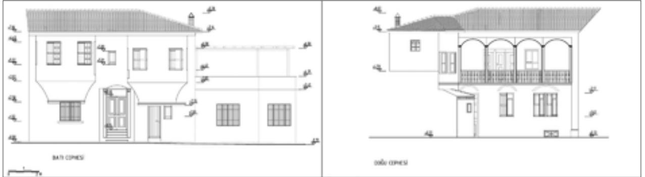
Şekil 17: Restorasyon ön cephe ve arka cephe.
