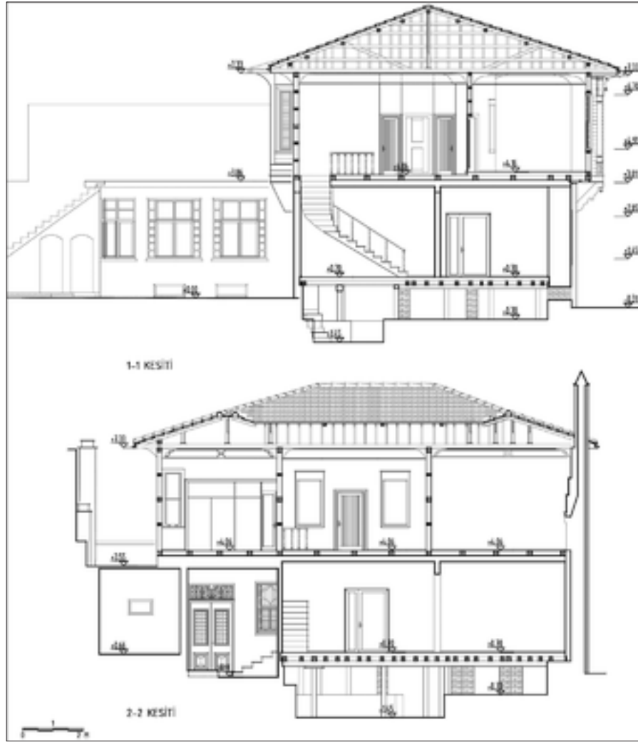
Şekil 14: Birinci dönem restitüsyon enine ve boyuna kesit.
