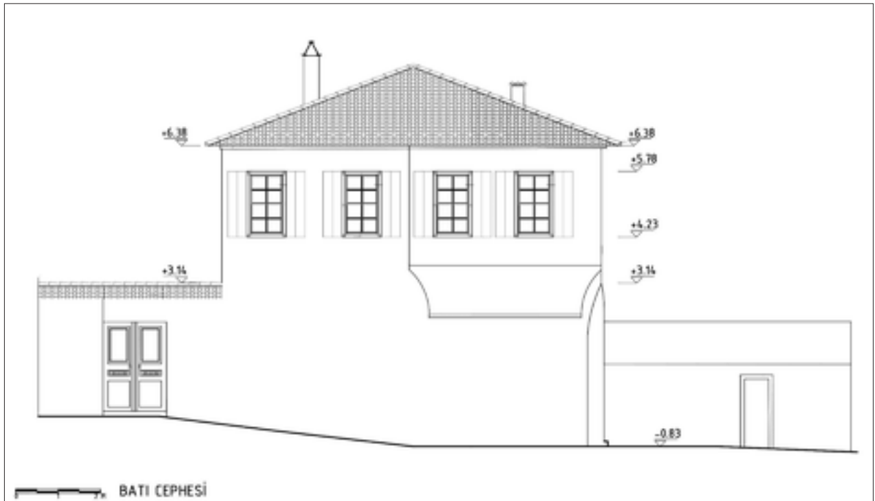
Şekil 21: Batı cephesi restorasyon önerisi.
