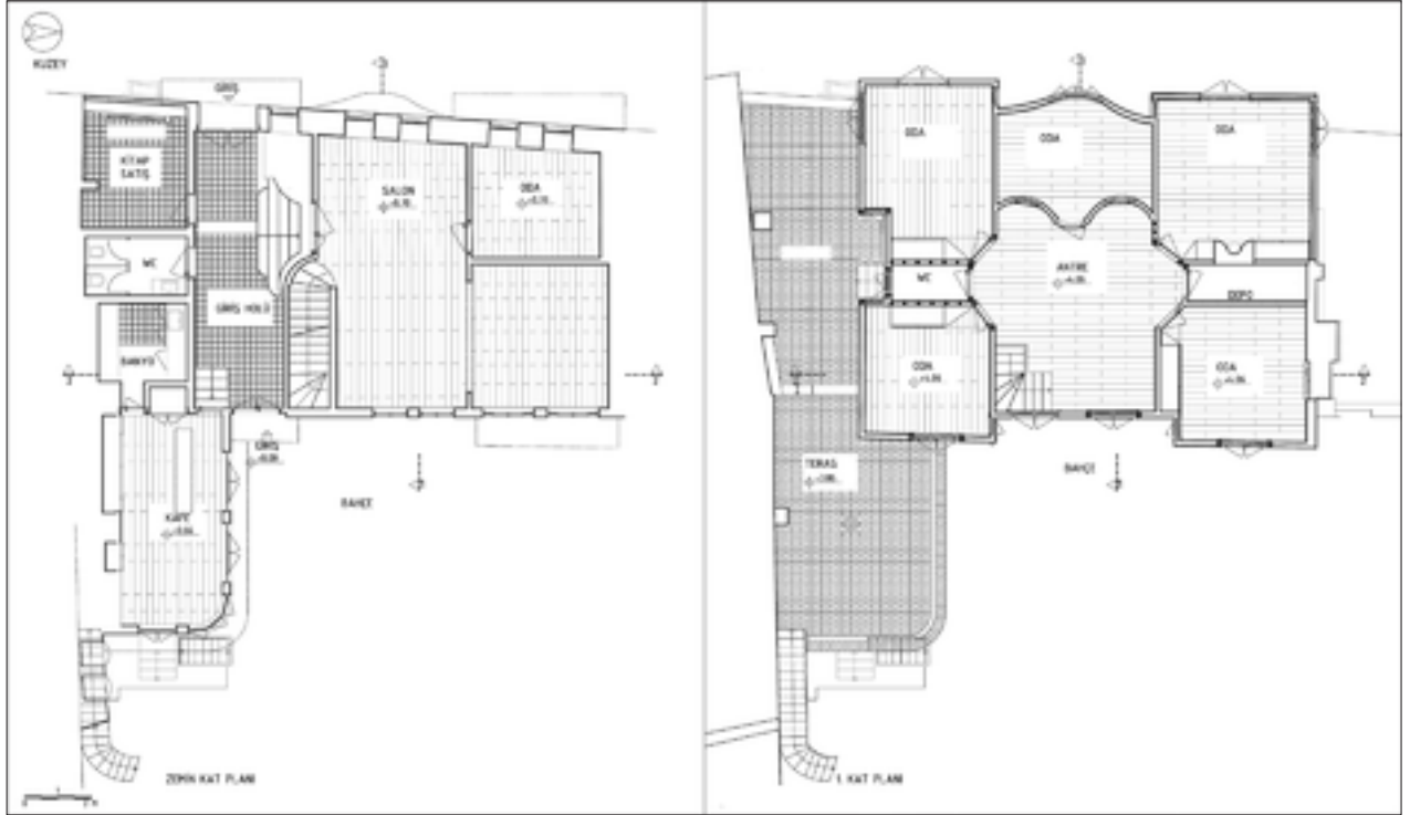
Şekil 16: Restorasyon kat planları.
