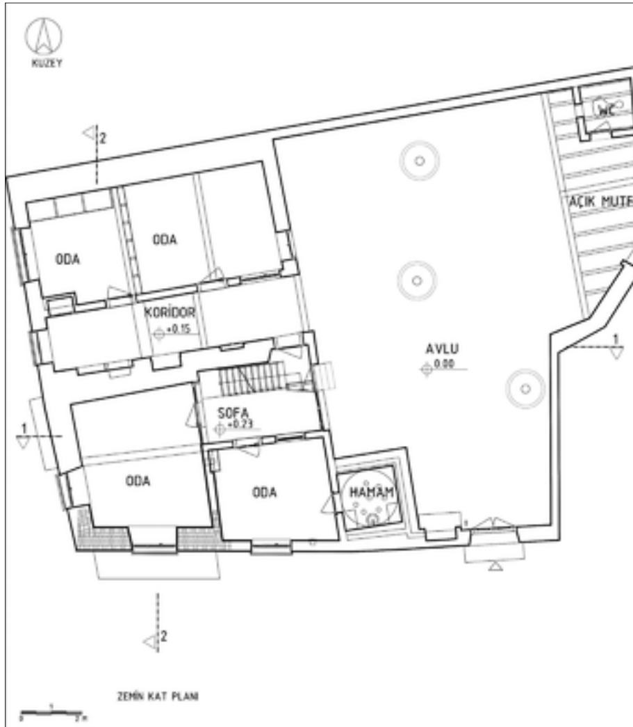
Şekil 9: Zemin kat döşeme planı.
