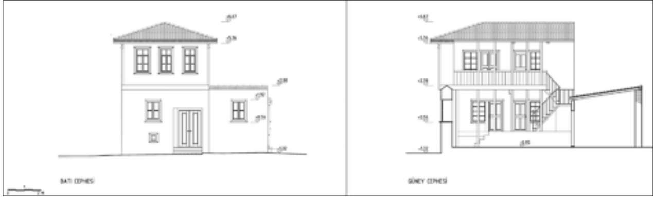
Şekil 23: Ön ve güney cephe restorasyonu.
