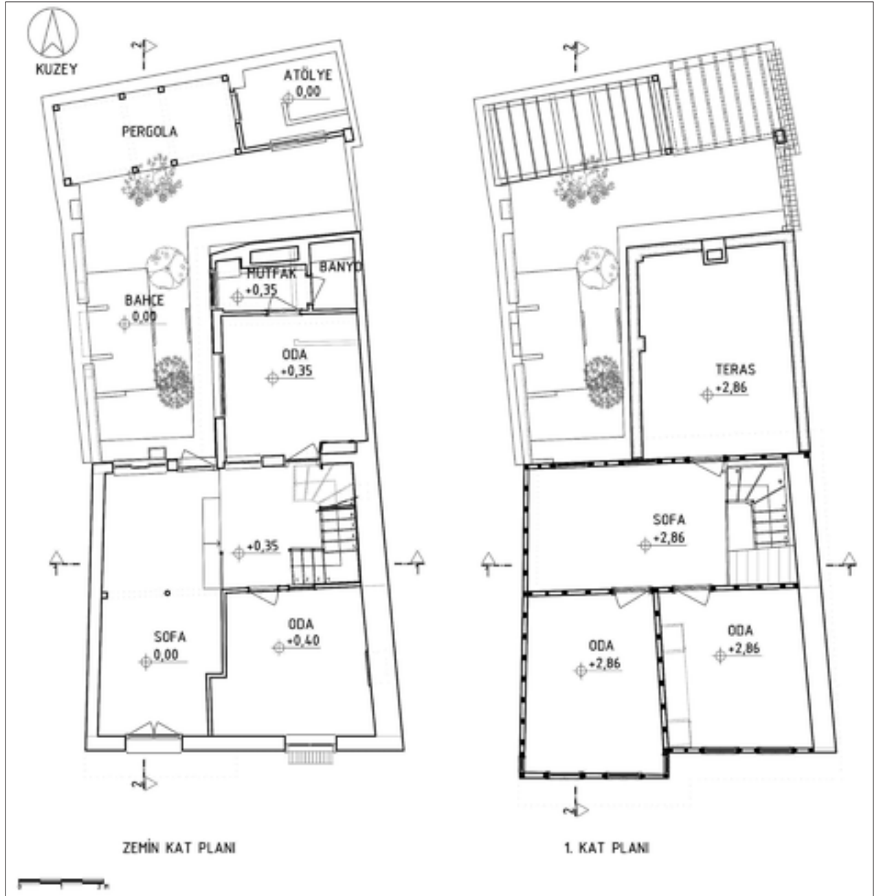
Şekil 9: Restorasyon zemin ve 1. kat planı önerisi.
